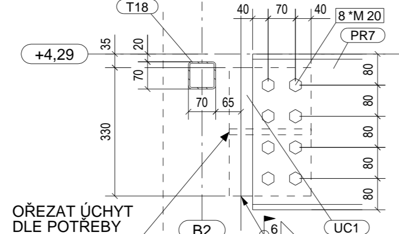
Řez B - B 1:10
