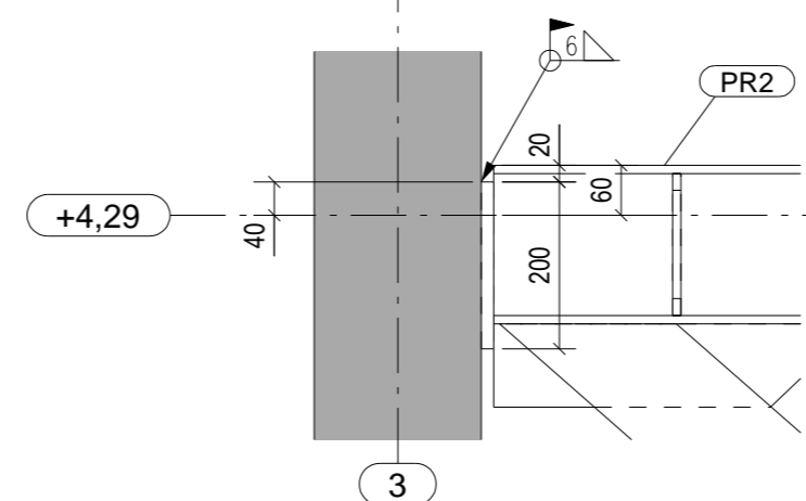
Řez C - C 1:10
