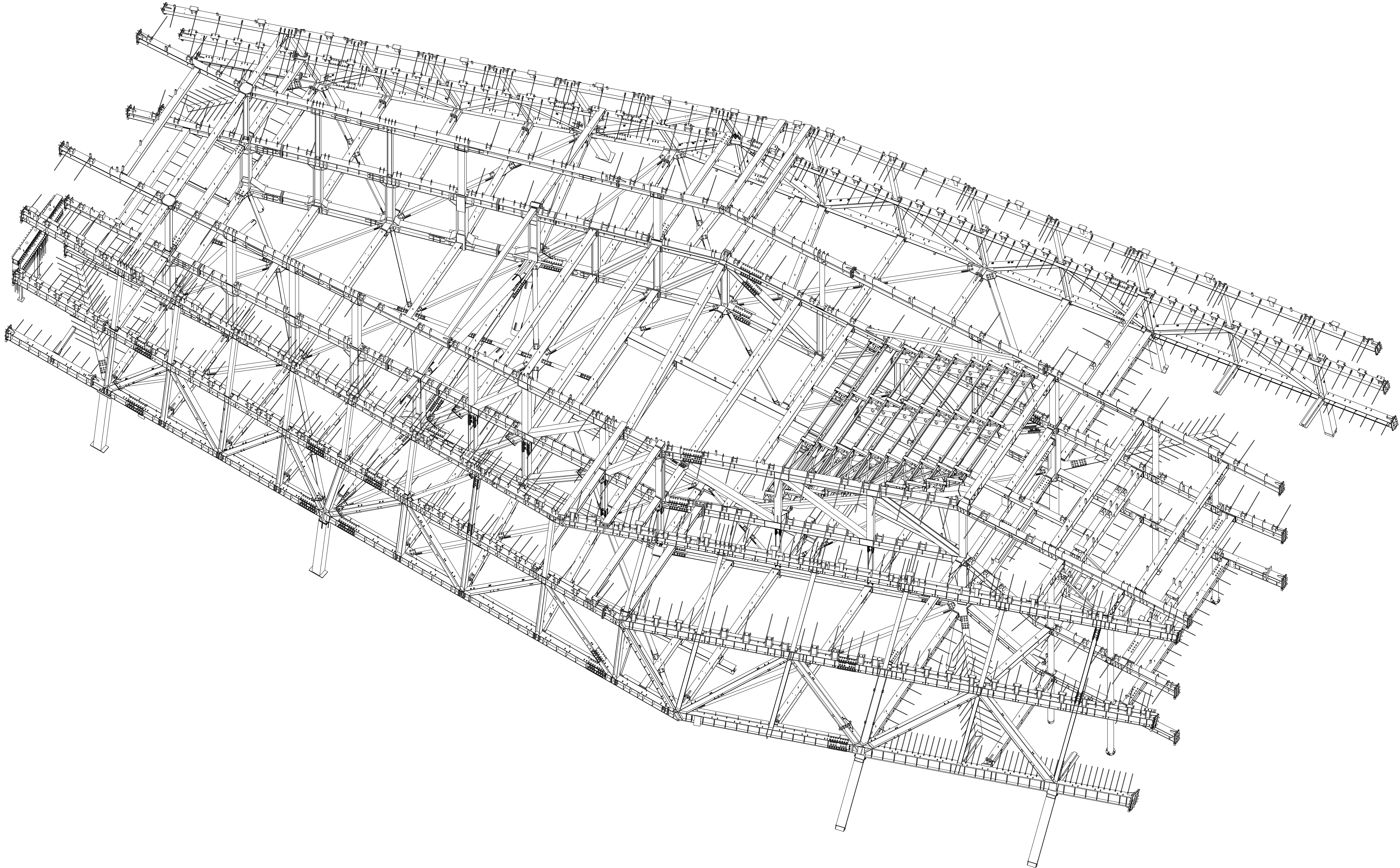
3D AANZICHT DAK/BRUG 1:65
