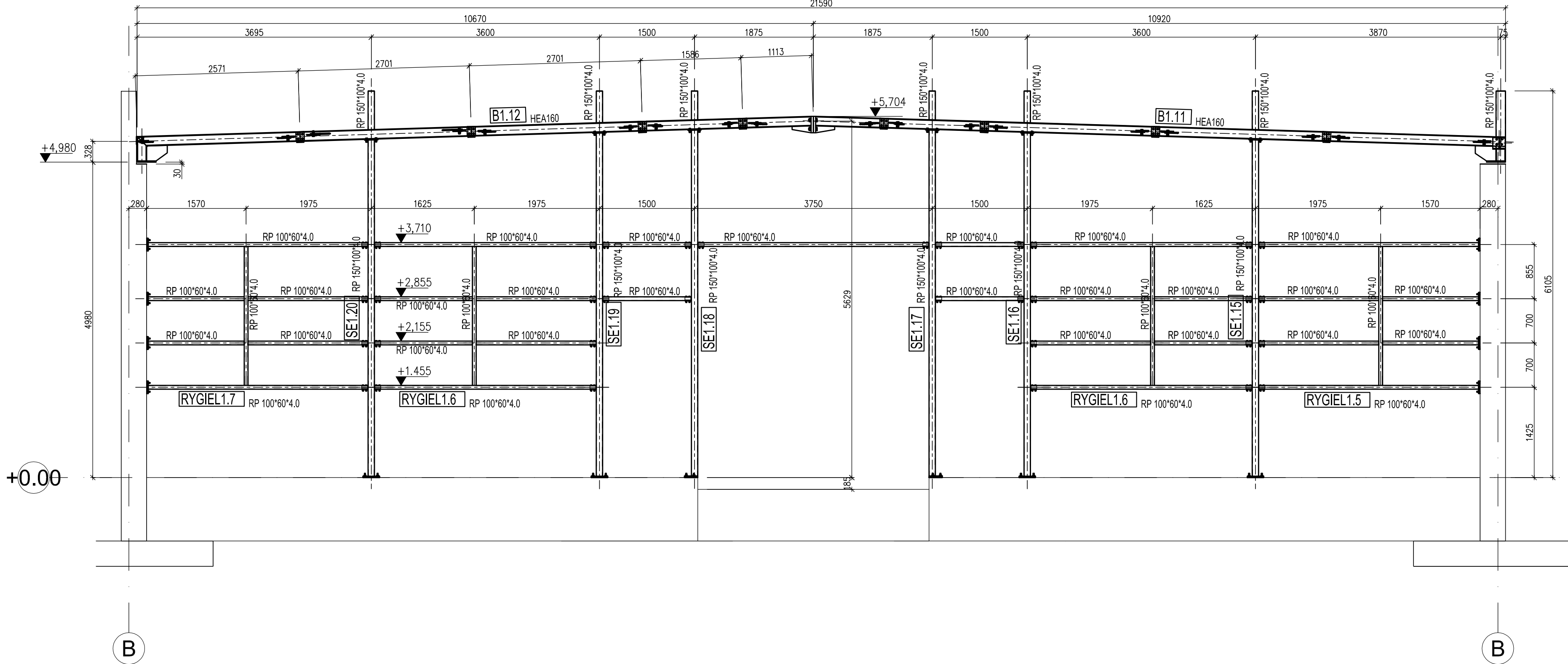
PRZĘKRÓJ 2.2-2.2 1:50
