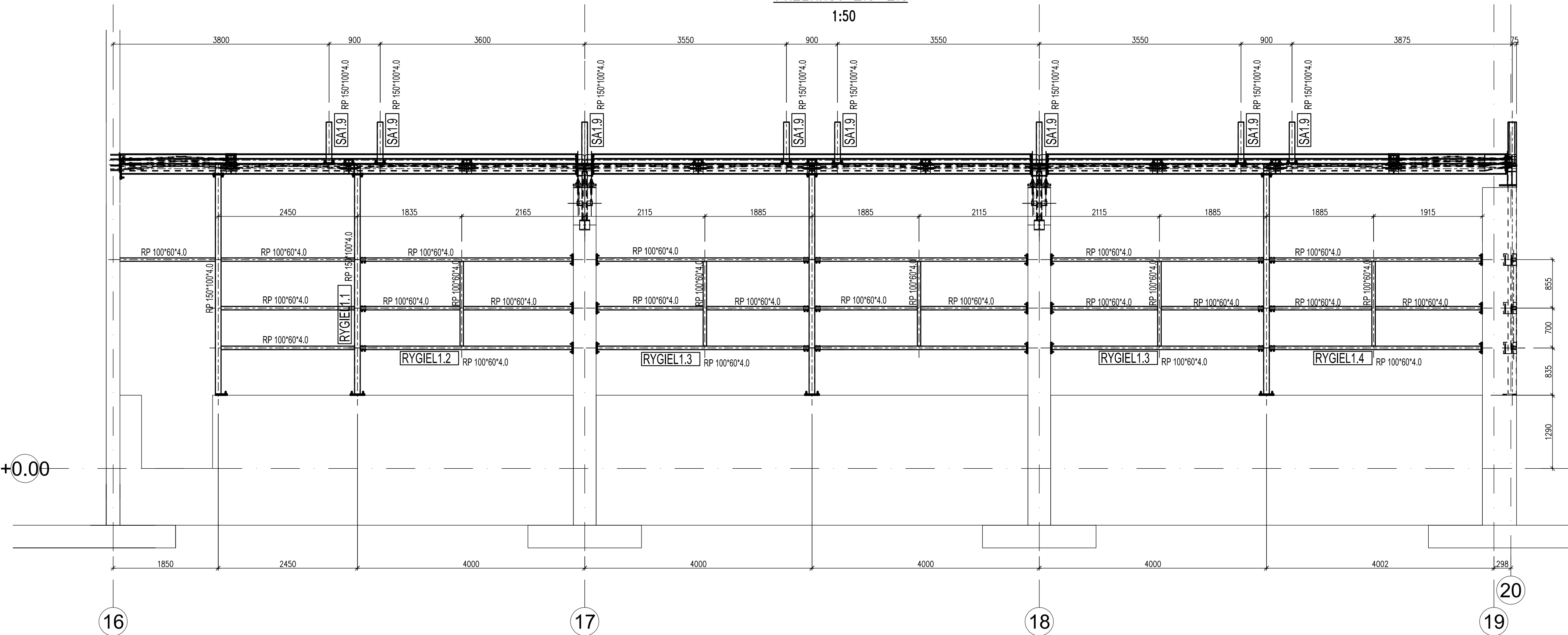
PRZĘKRÓJ 2.3-2.3 1:50
