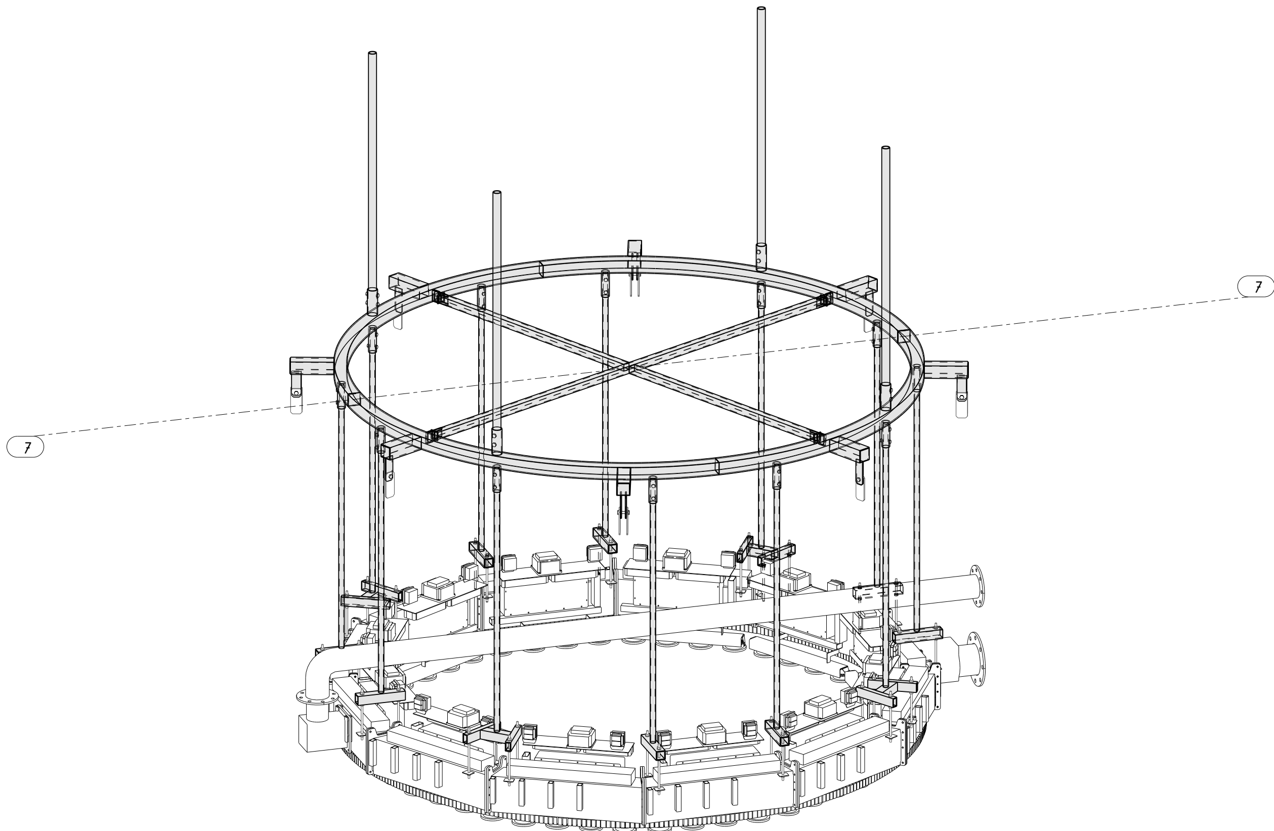
Rzut aksonometryczny konstrukcji podwieszającej i Flashwalla 1:20
