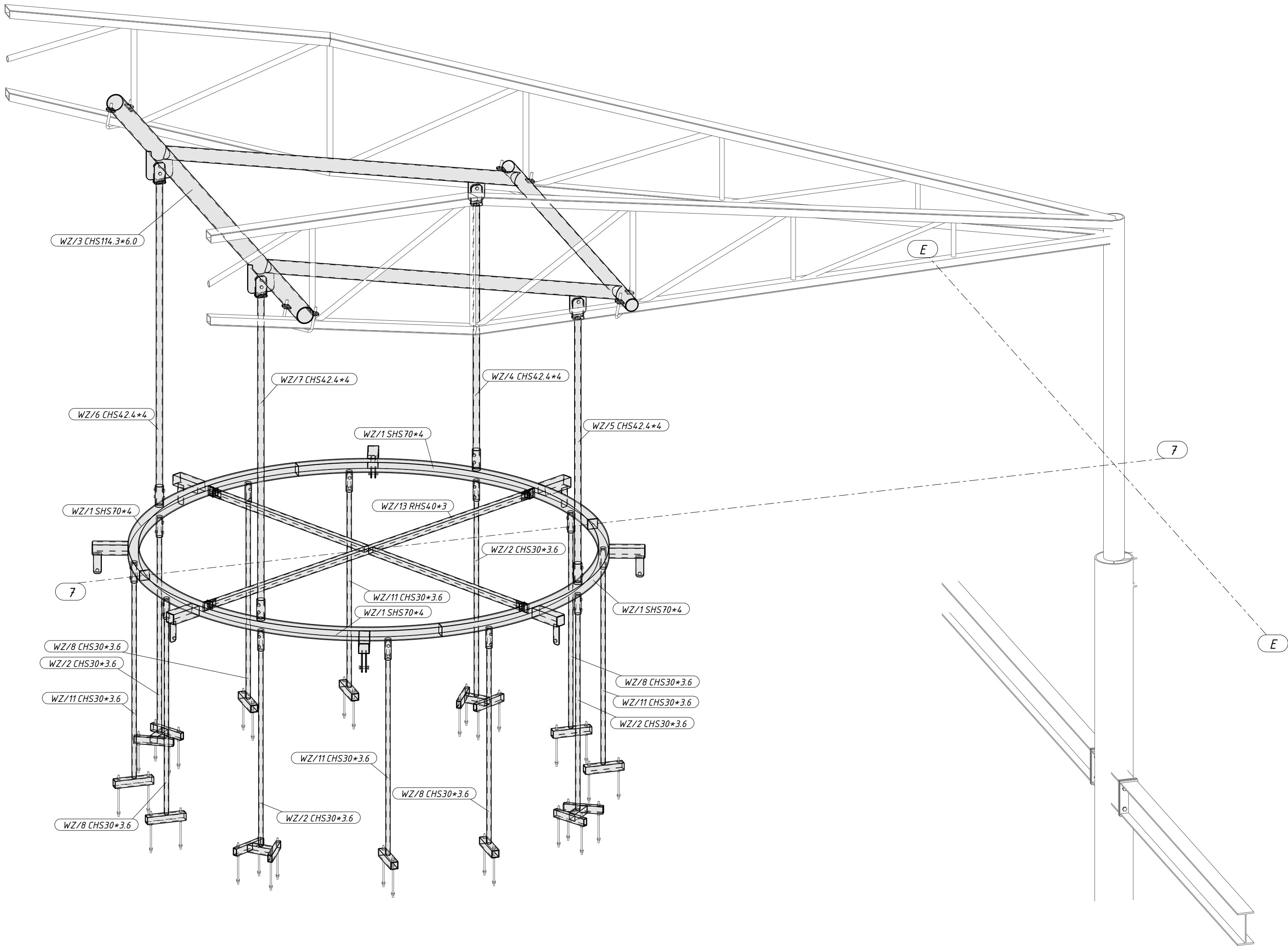
Rzut aksonometryczny konstrukcji podwieszającej 1:20
