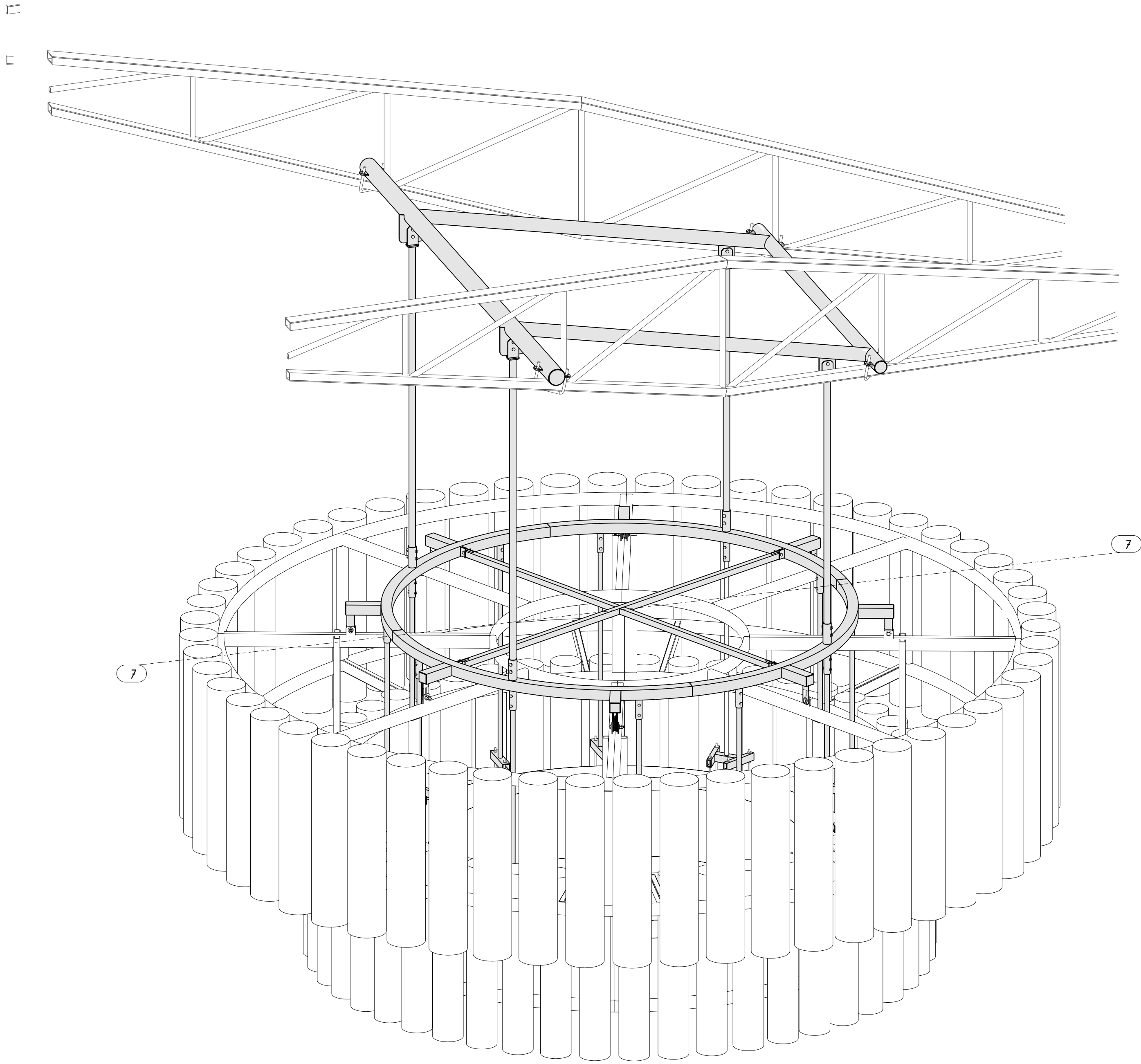
Rzut aksonometryczny konstrukcji podwieszającej i żyrandola 1:20
