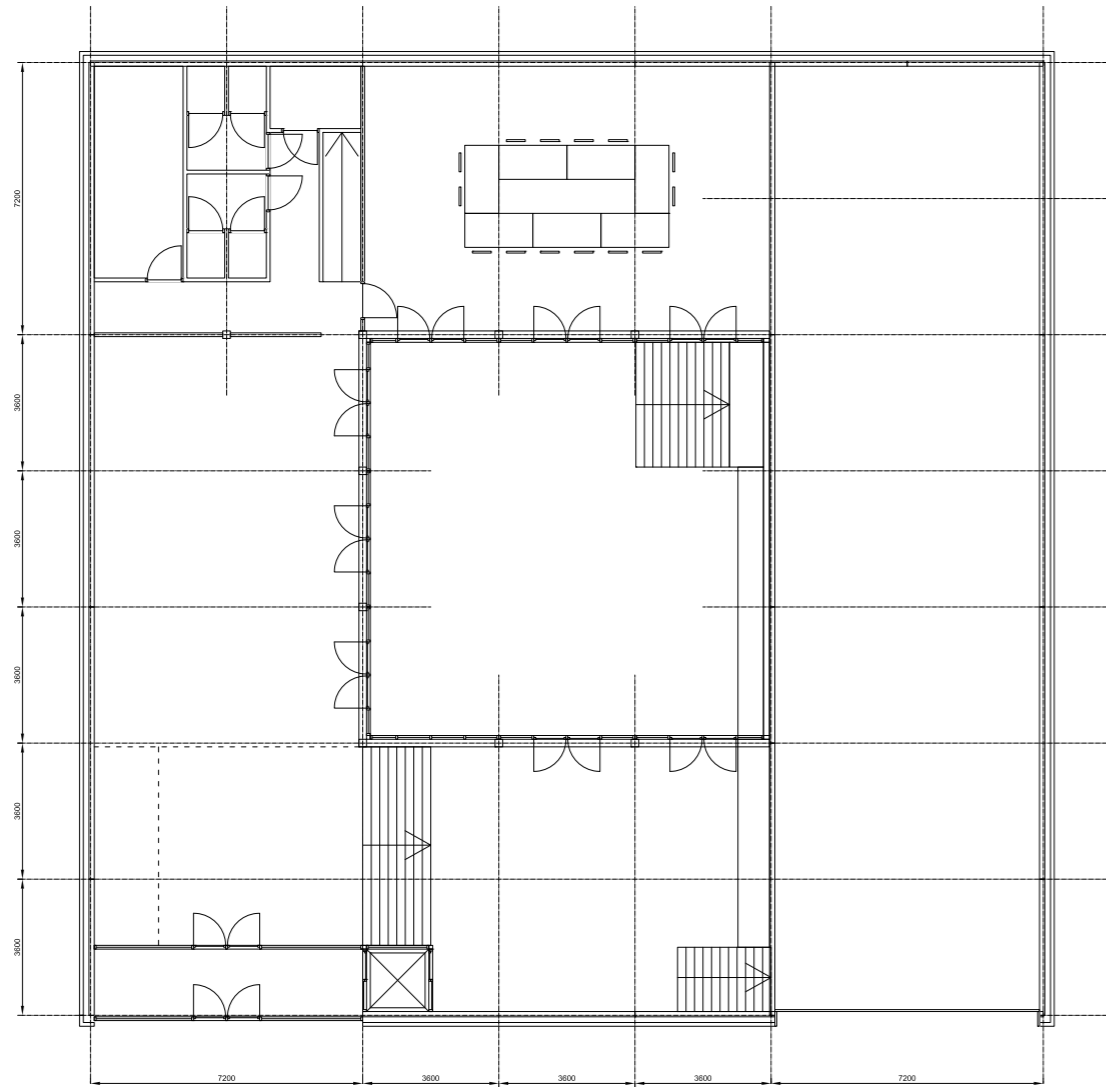
BEGANE GROND
