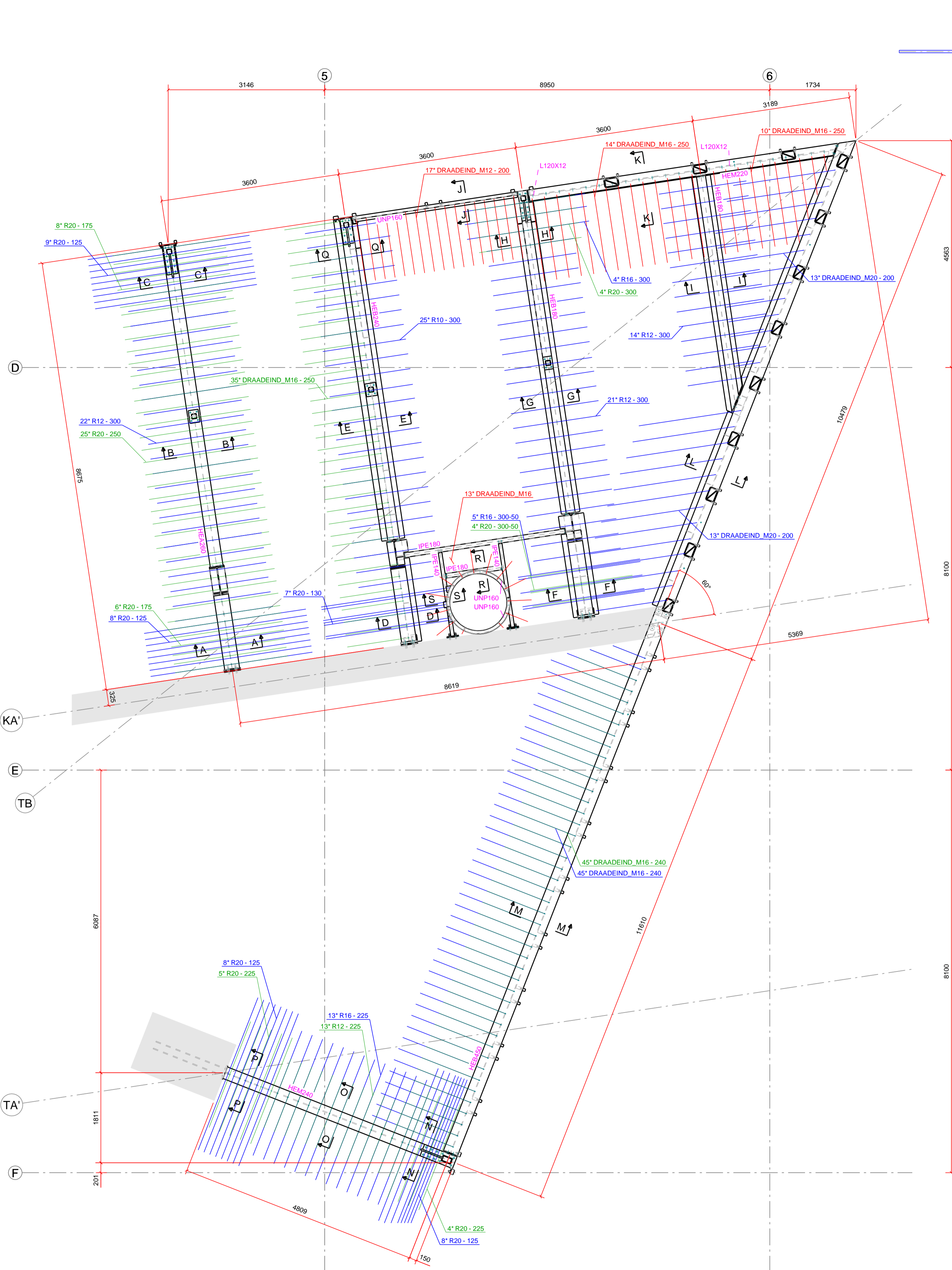
Overzicht 02 tweede verdieping +8800 1:50
