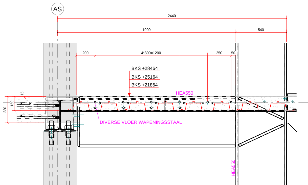
DOORSNEDE A-A 1:15
