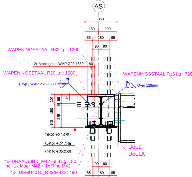
DOORSNEDE B-B 1:15
