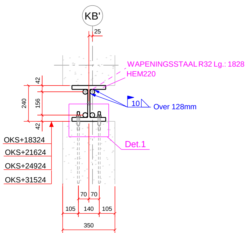
DOORSNEDE A-A 1:15
