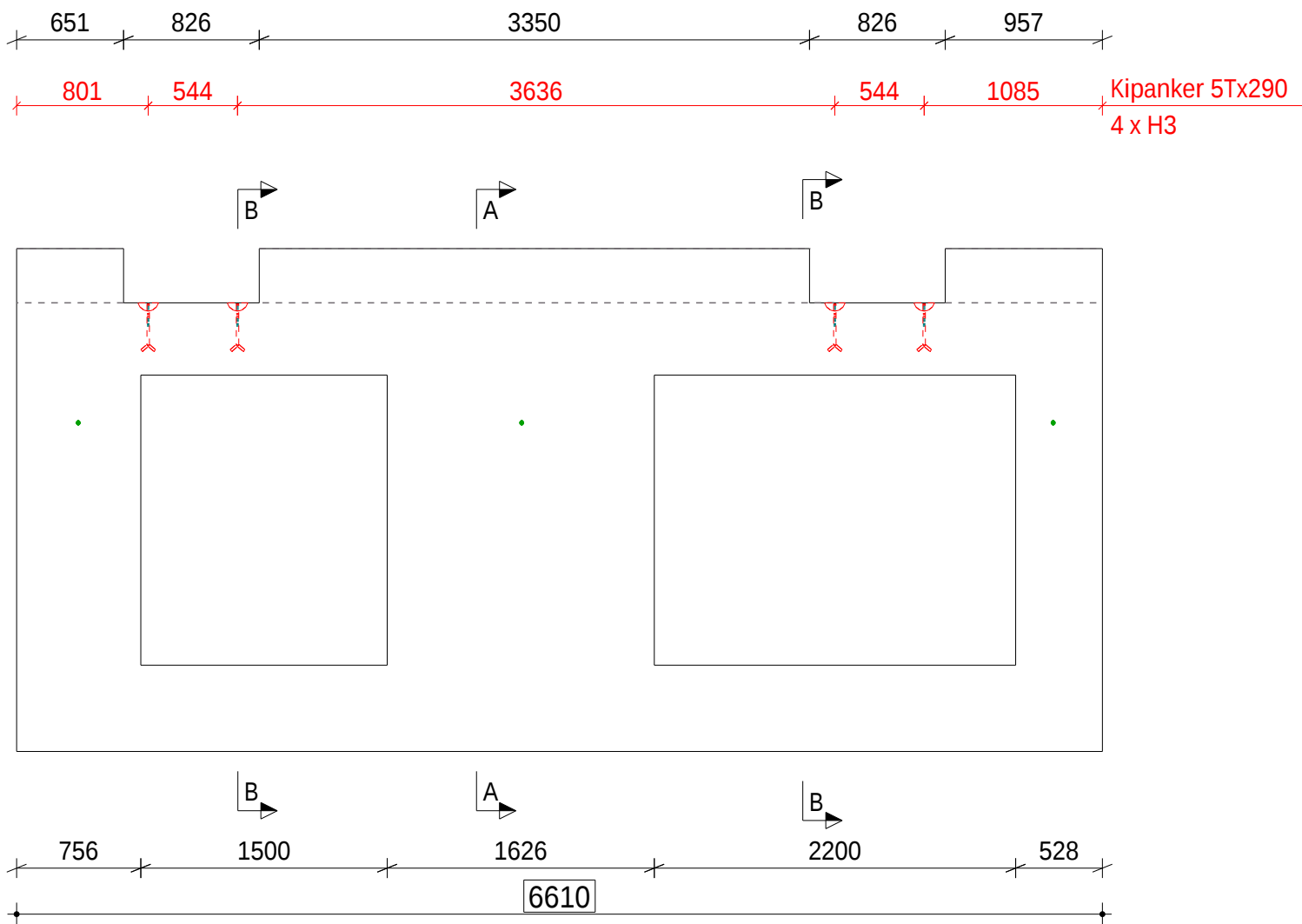
Vue coté taloche / Afgestreken zijde
