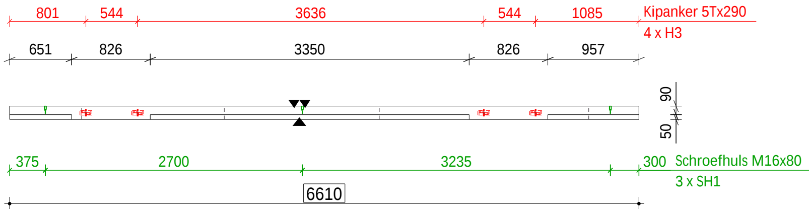
Vue dessus / Bovenaanzicht
