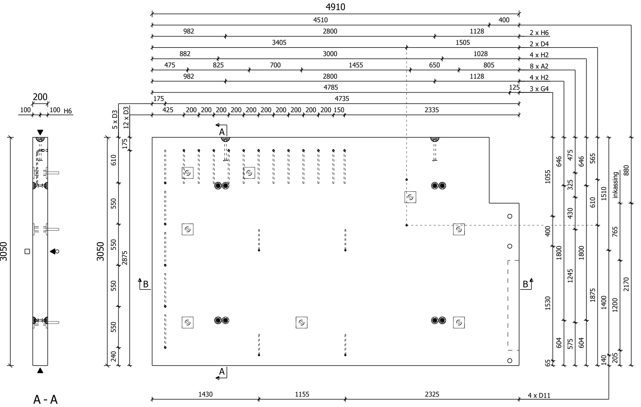
Vooraanzicht (stortzijde)
