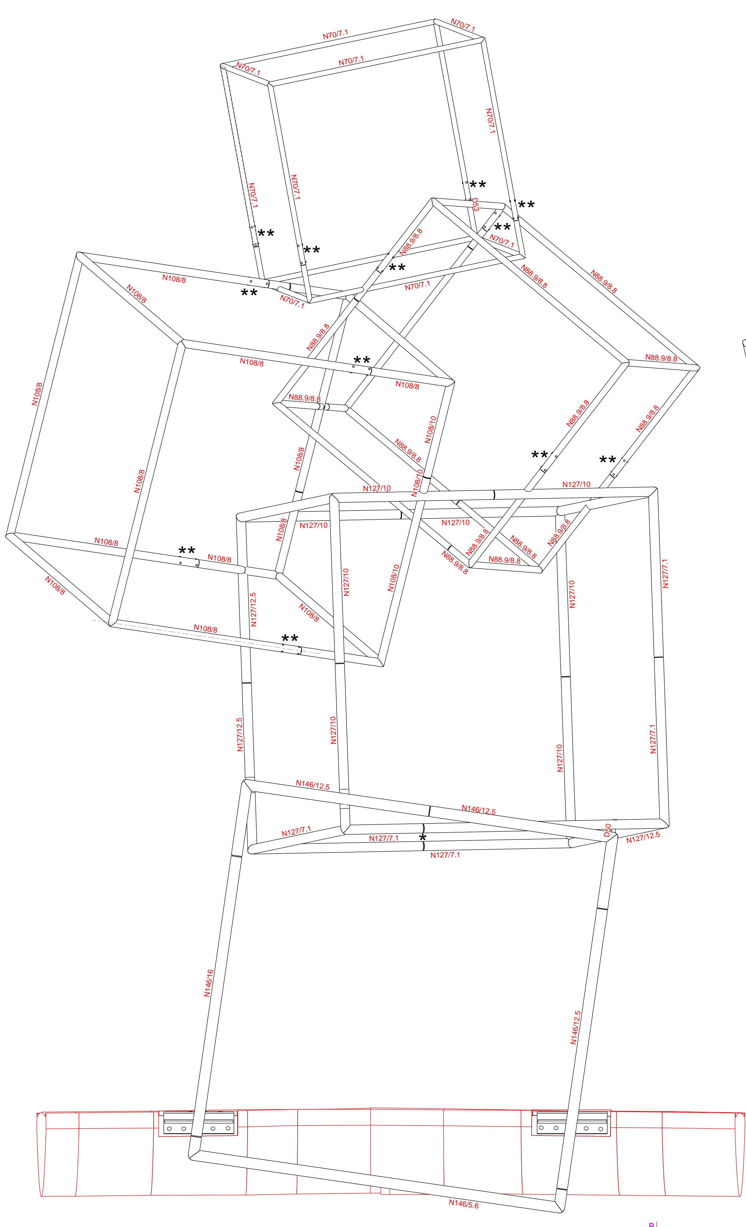
Voor aanzicht
