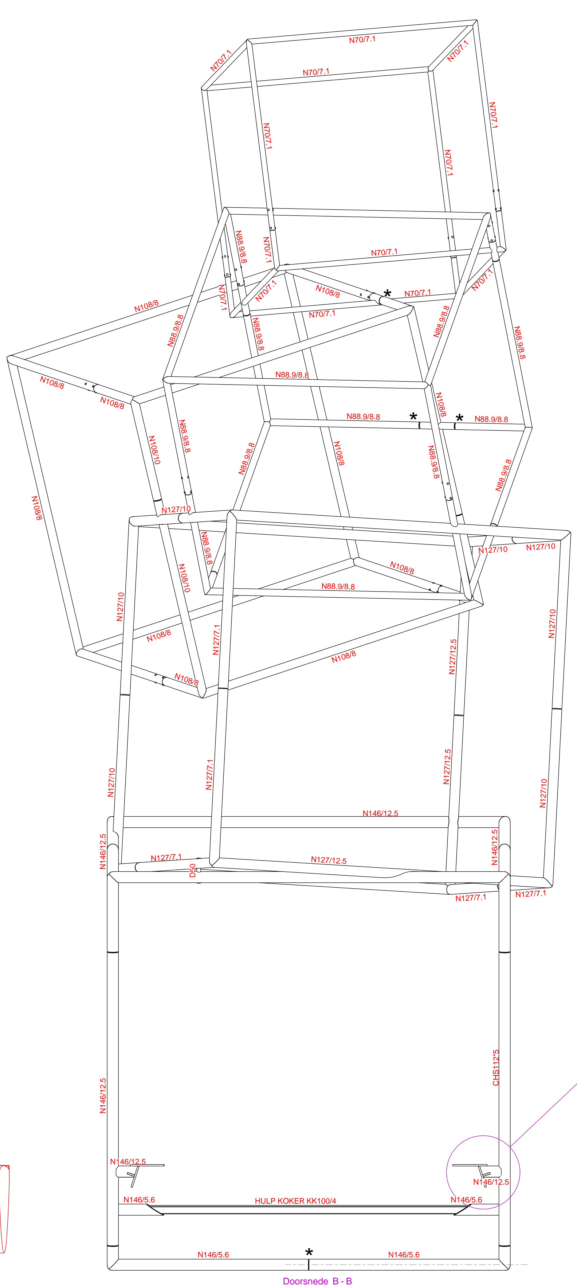
Doorsnede B - B
