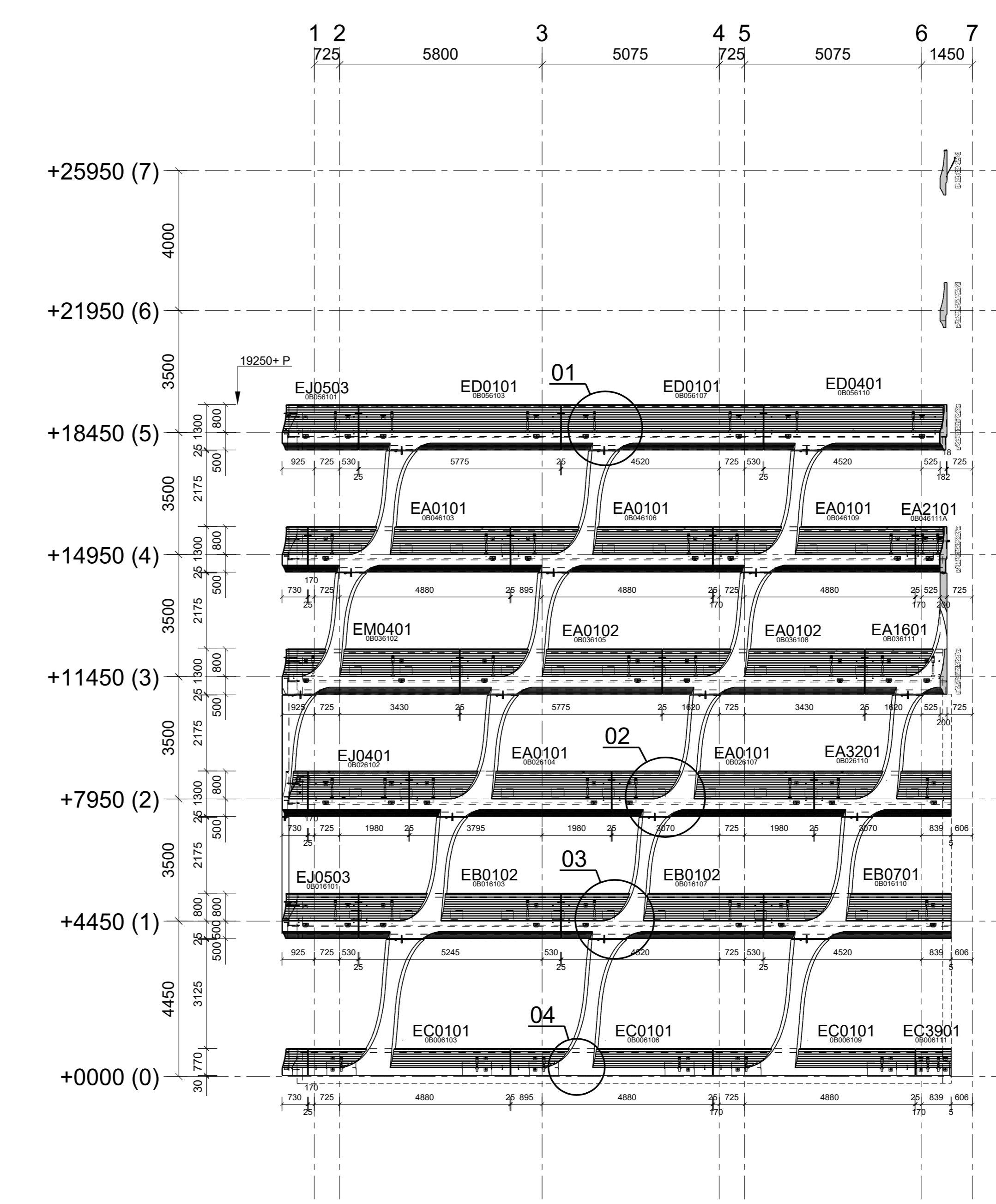
Achse A6
