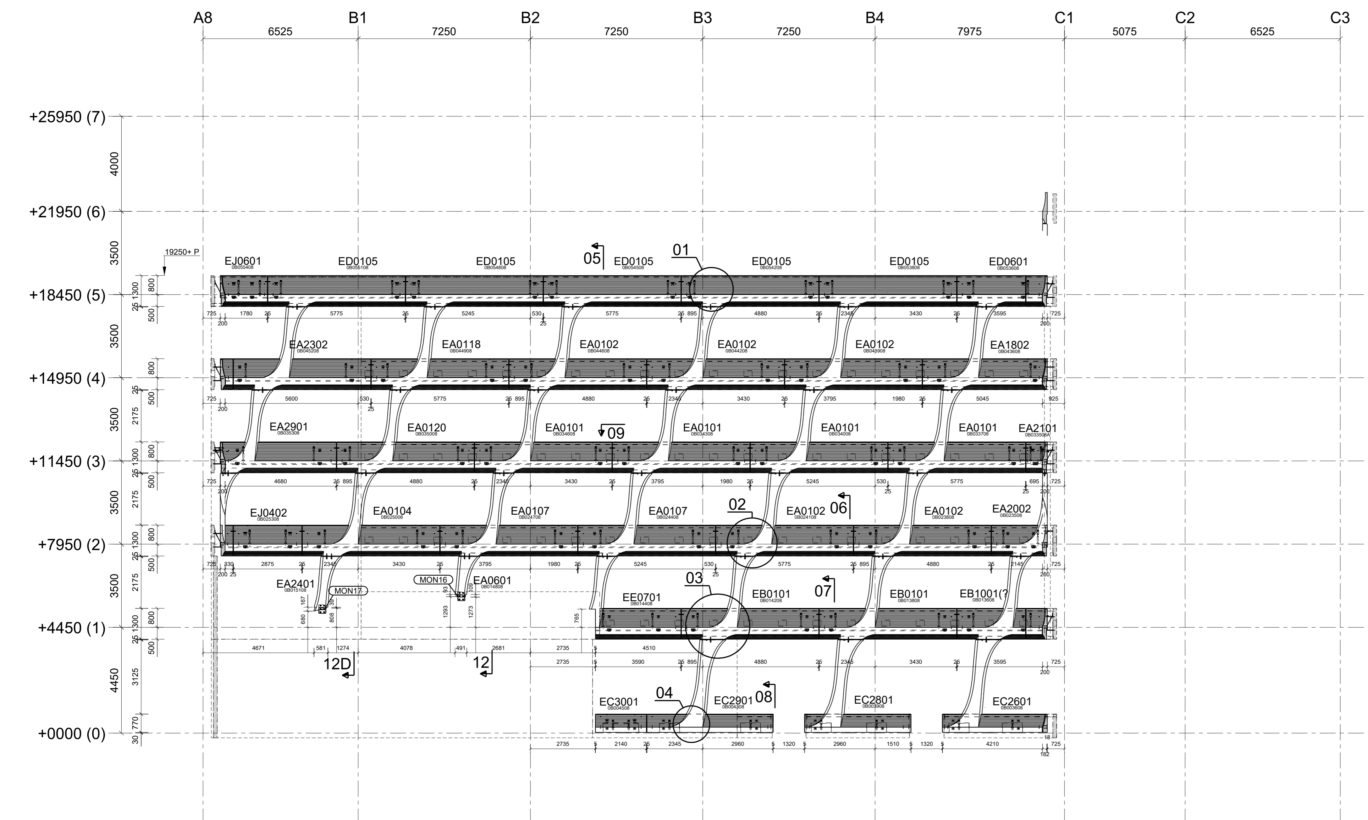
Achse 5
