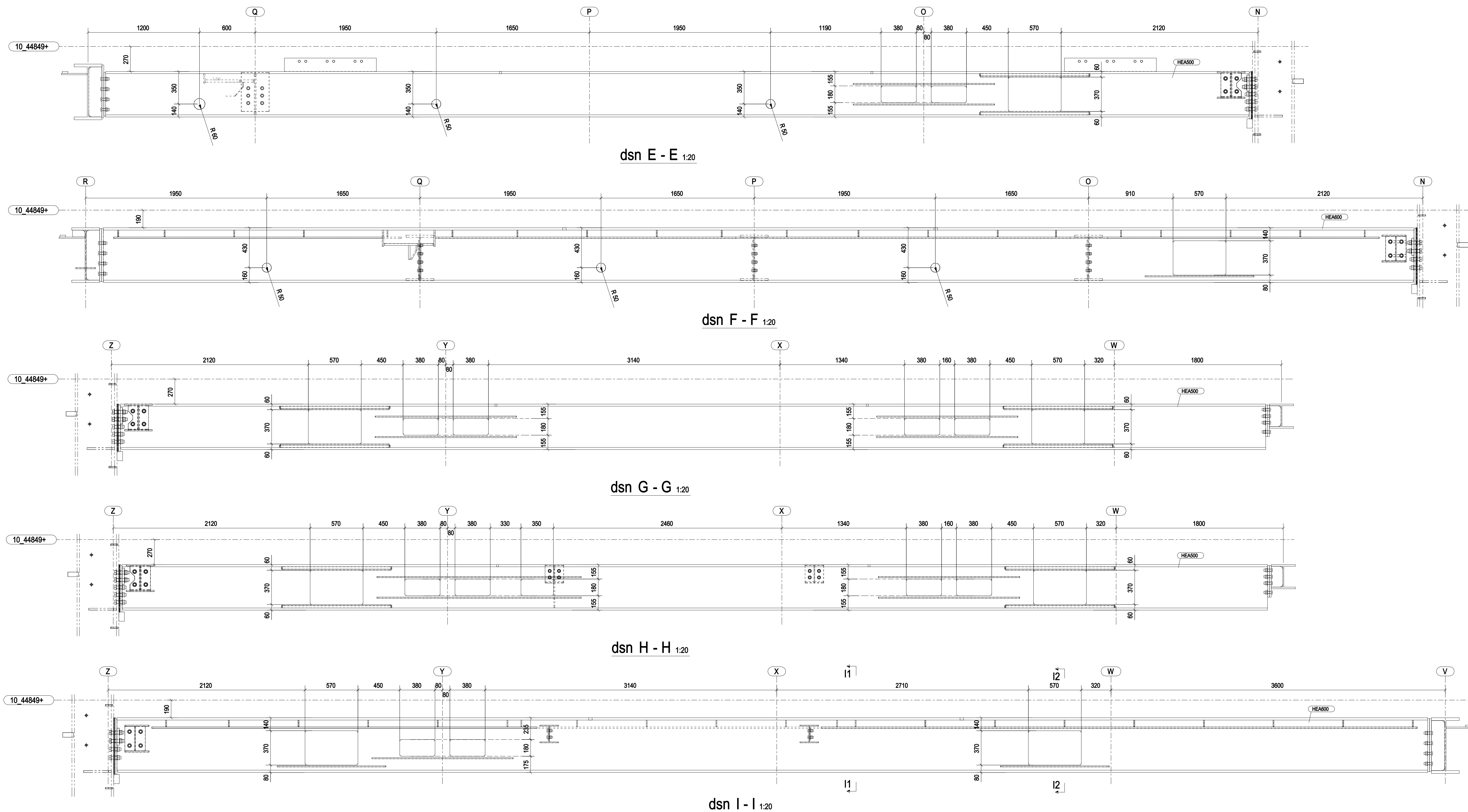
dsn I - I 1:20
