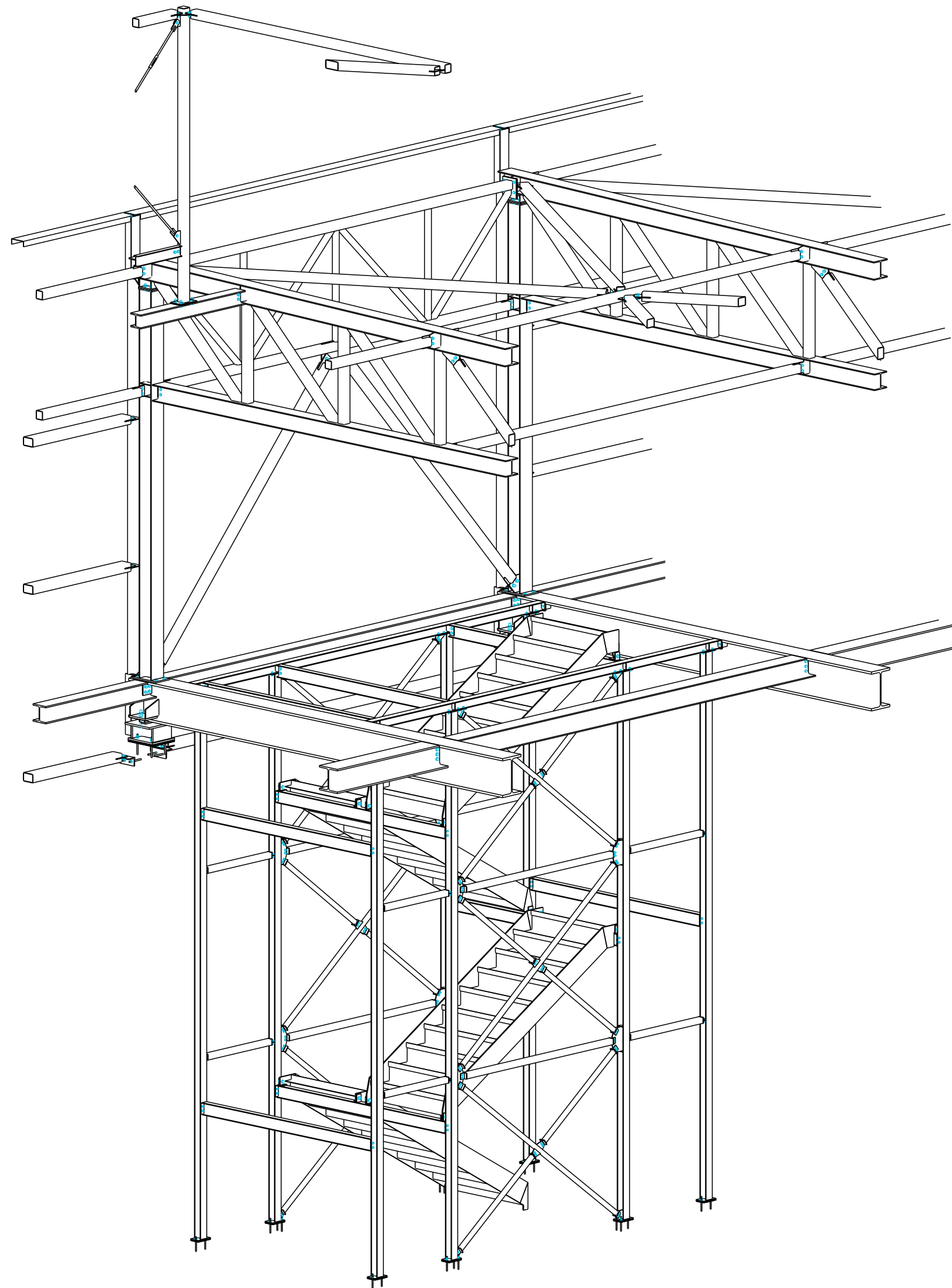
3D SCHODY MEZI OSAMI Y-Z 1:50
