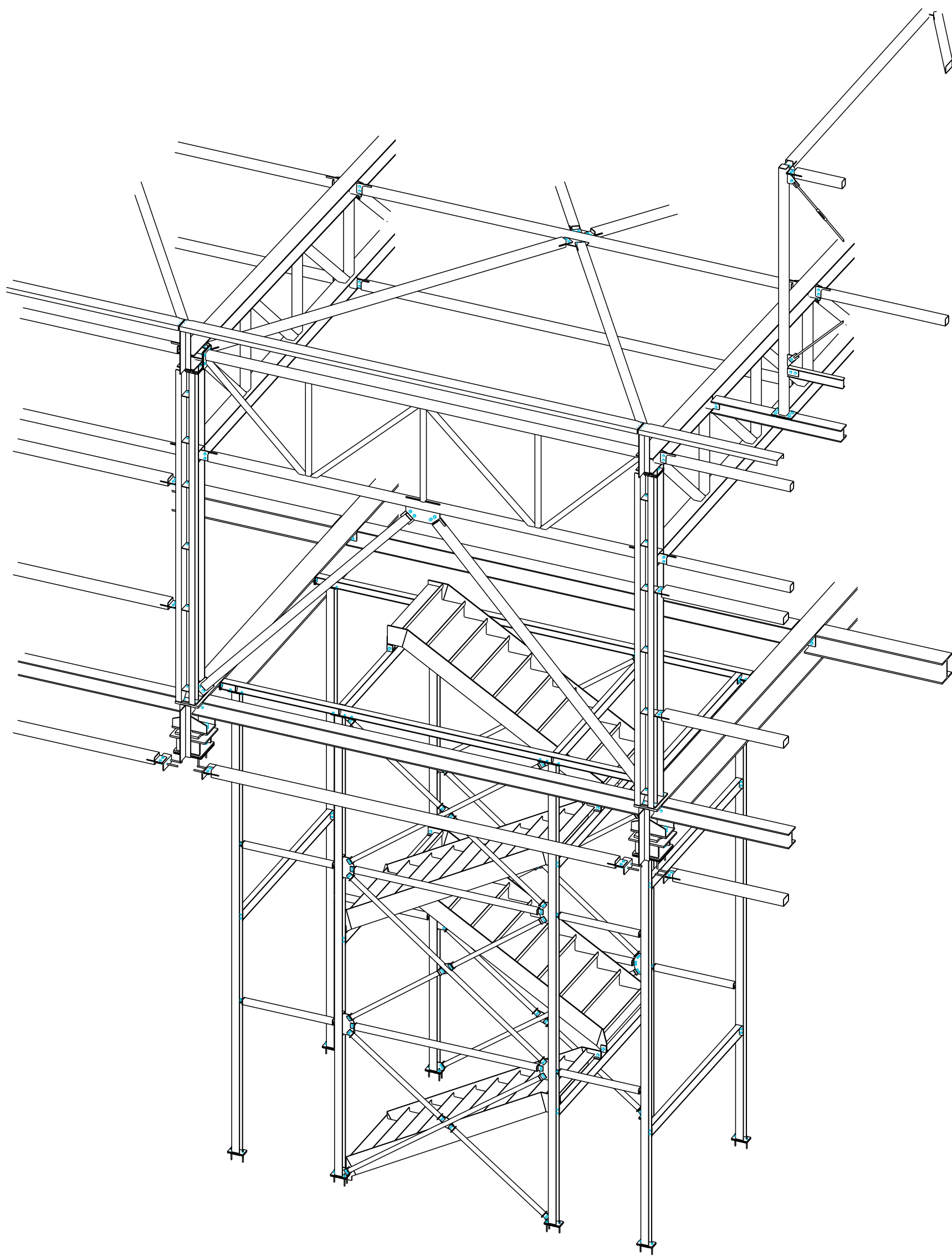
3D SCHODY MEZI OSAMI P-Q 1:50
