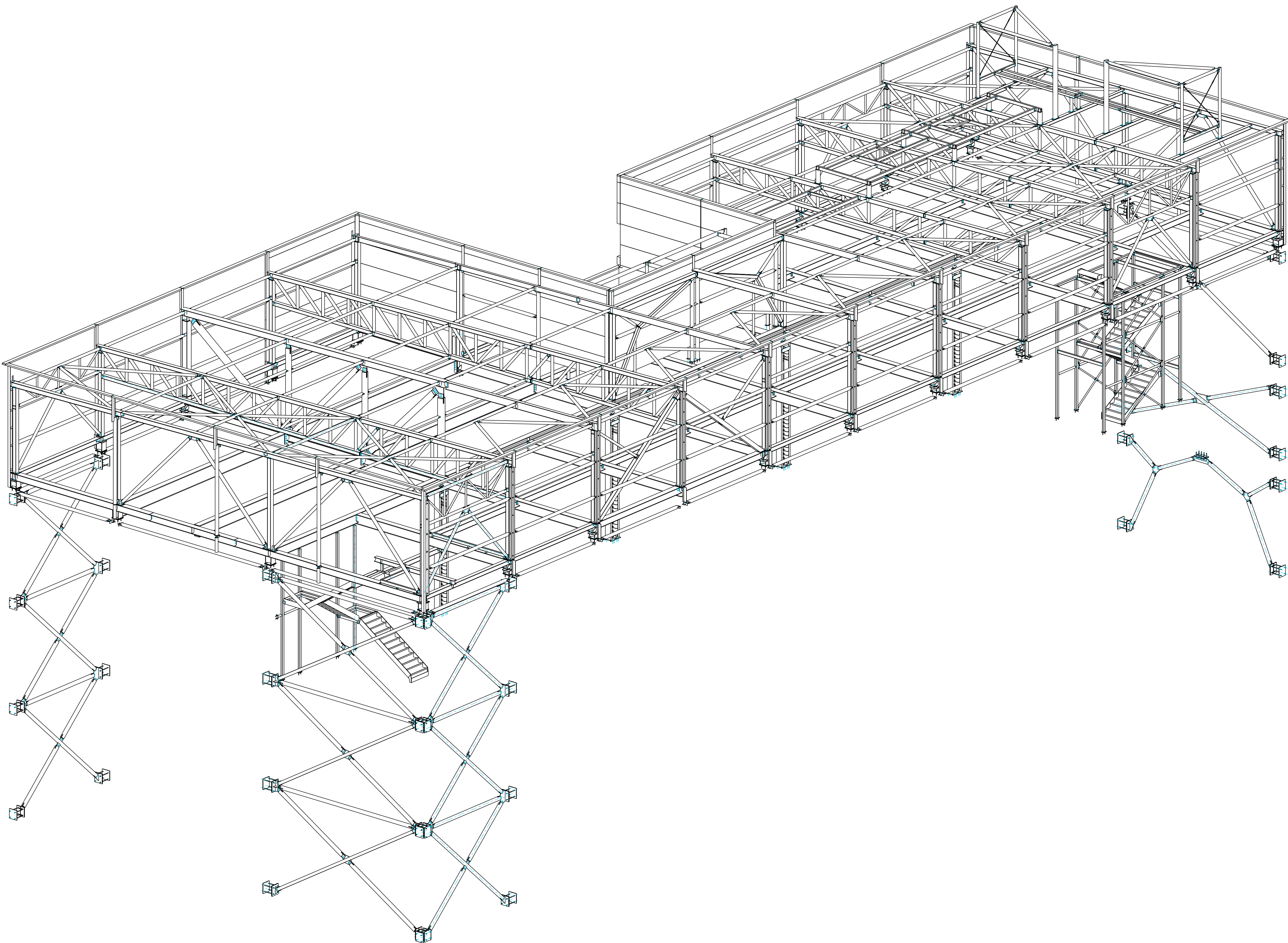
3D POHLED 1:100
