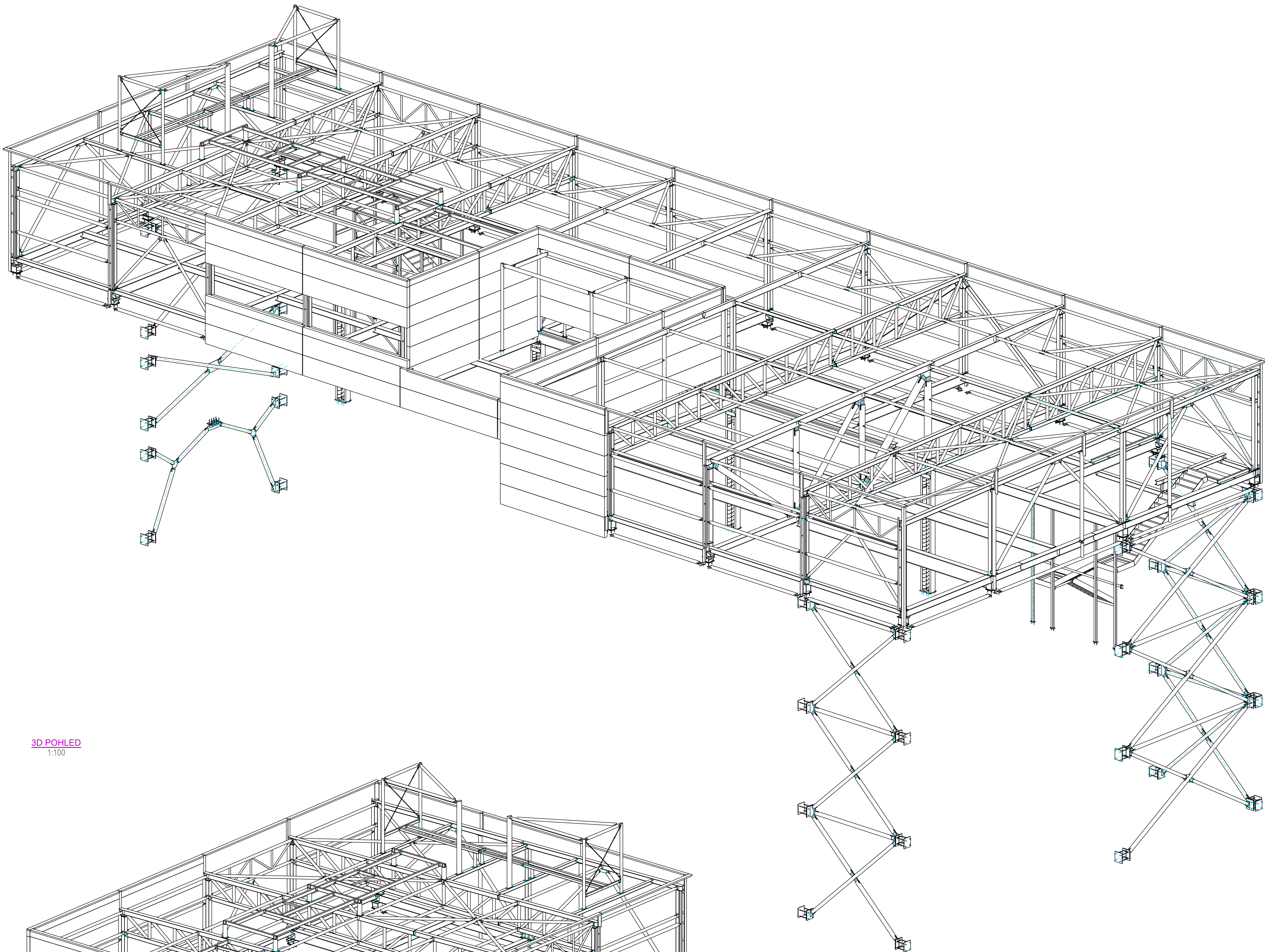
3D POHLED 1:100
