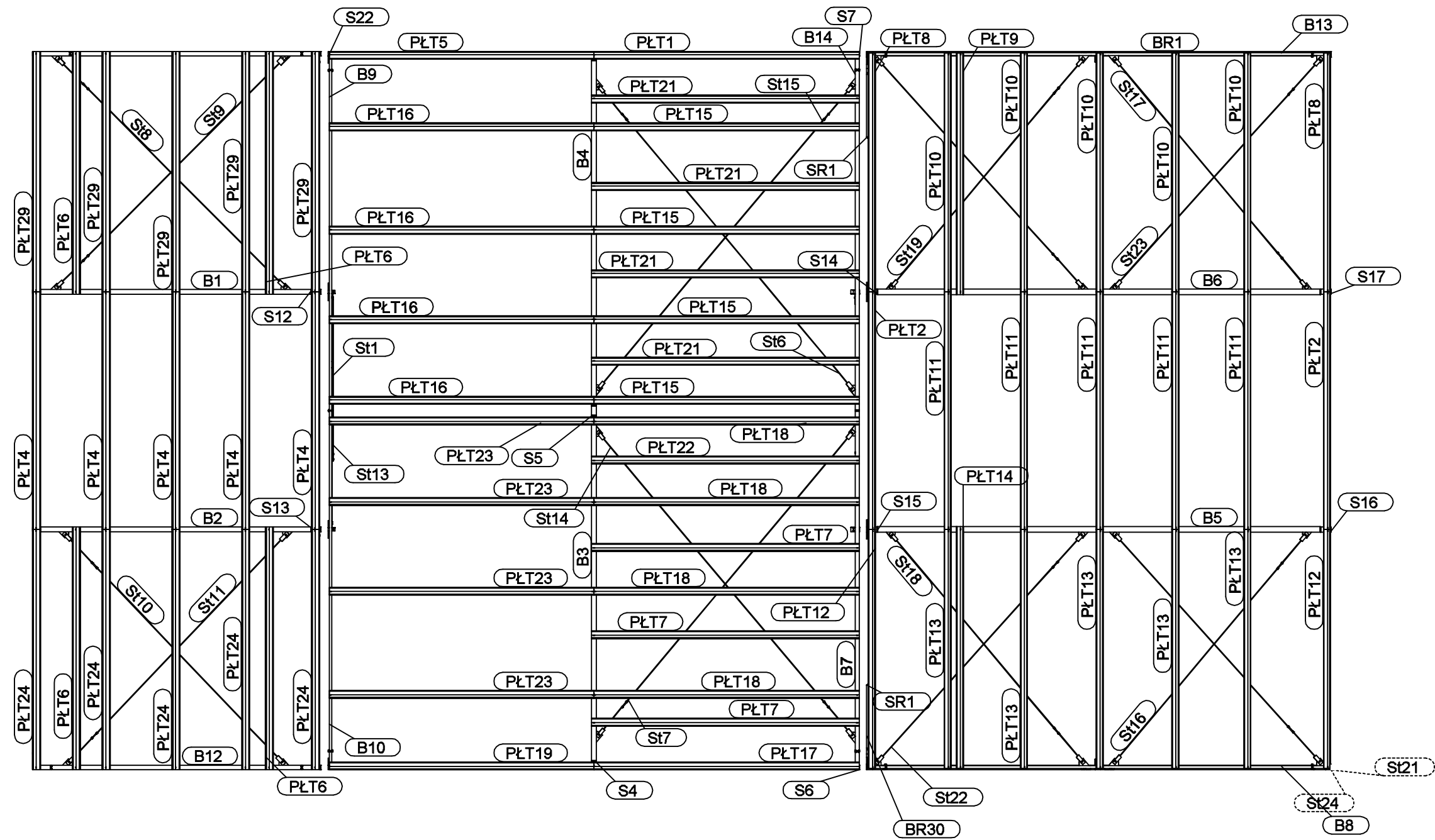
Rzut dachu 1:100
