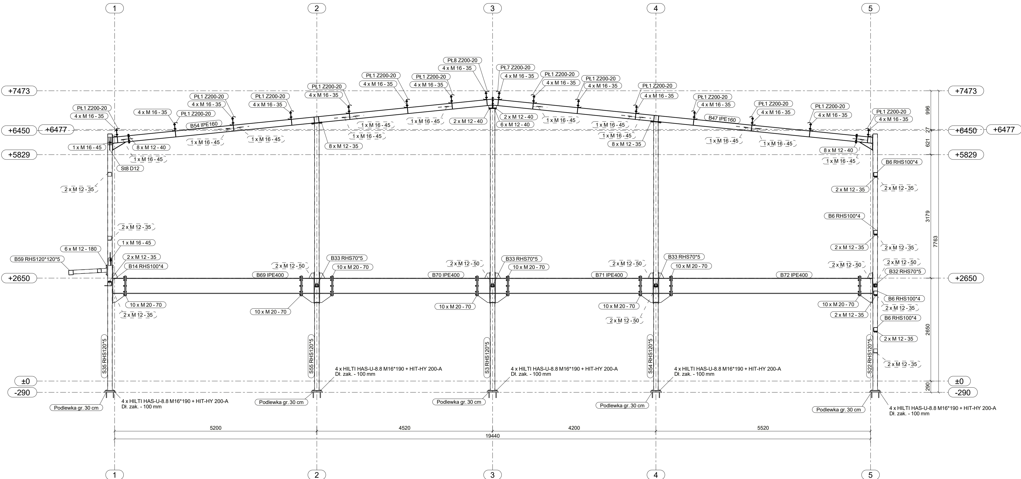
Przekrój w osi J 1:50
