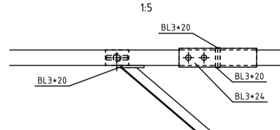
G - G 1:5
