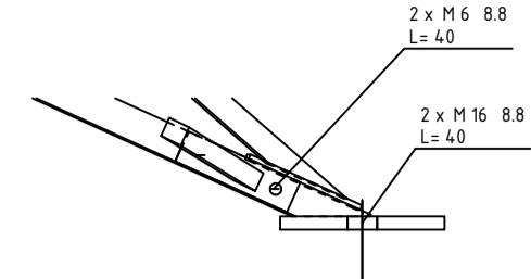
B - B 1:5
