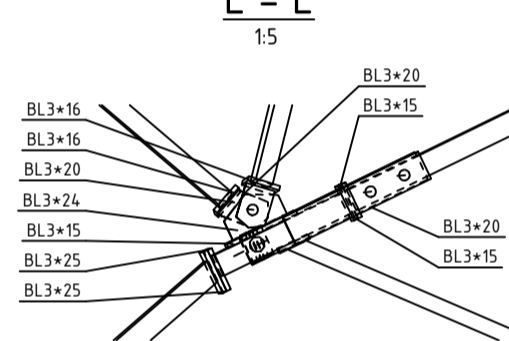
E - E 1:5
