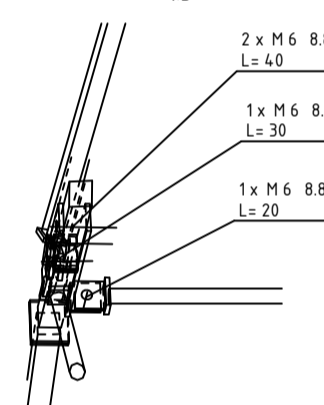
F - F 1:5
