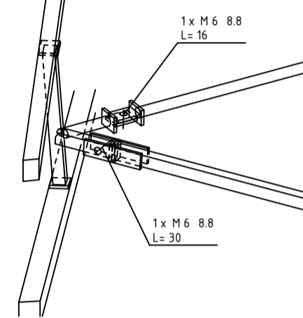
D - D 1:5
