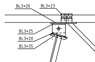
I - I 1:5
