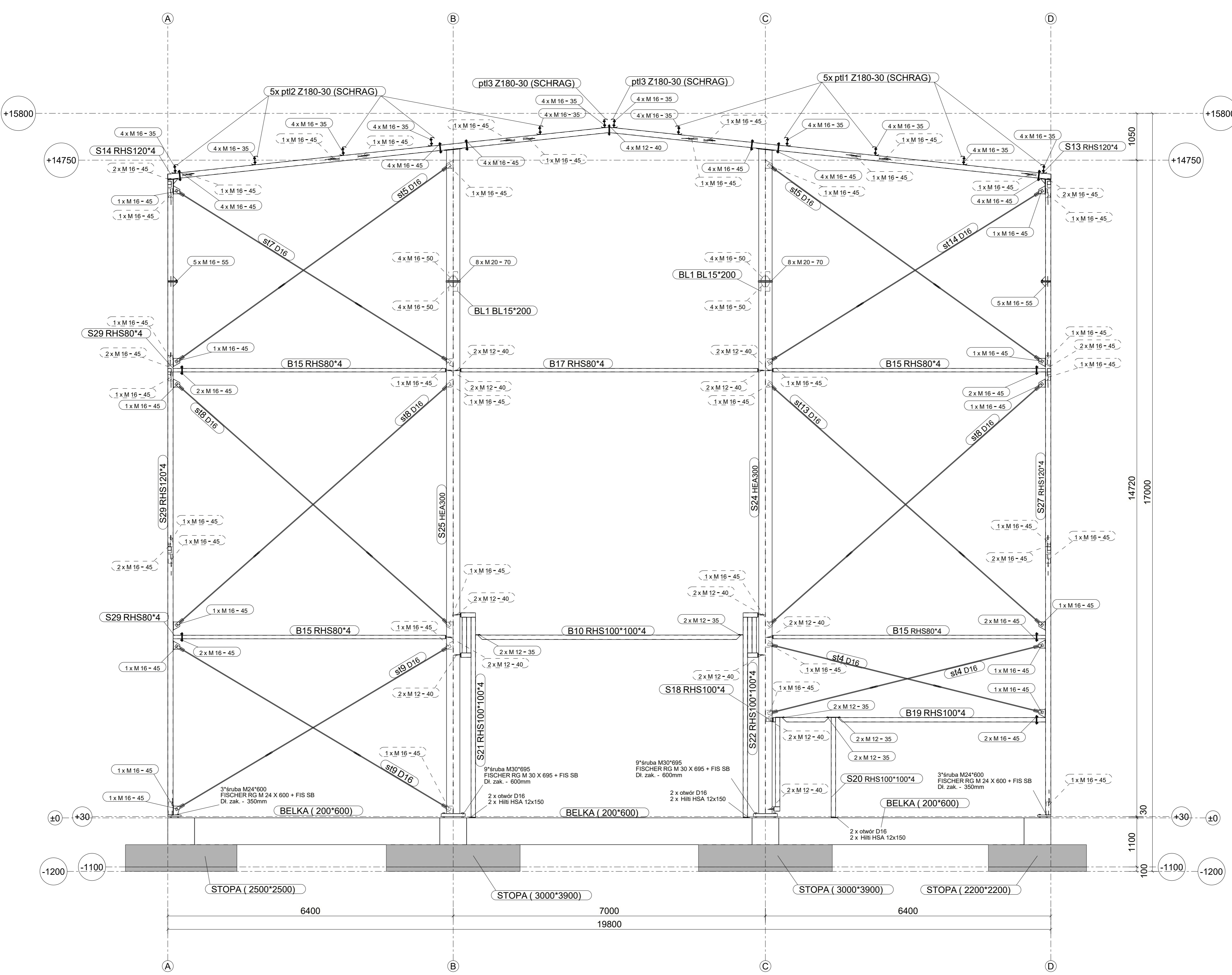
Przekrój w osi 1 1:50
