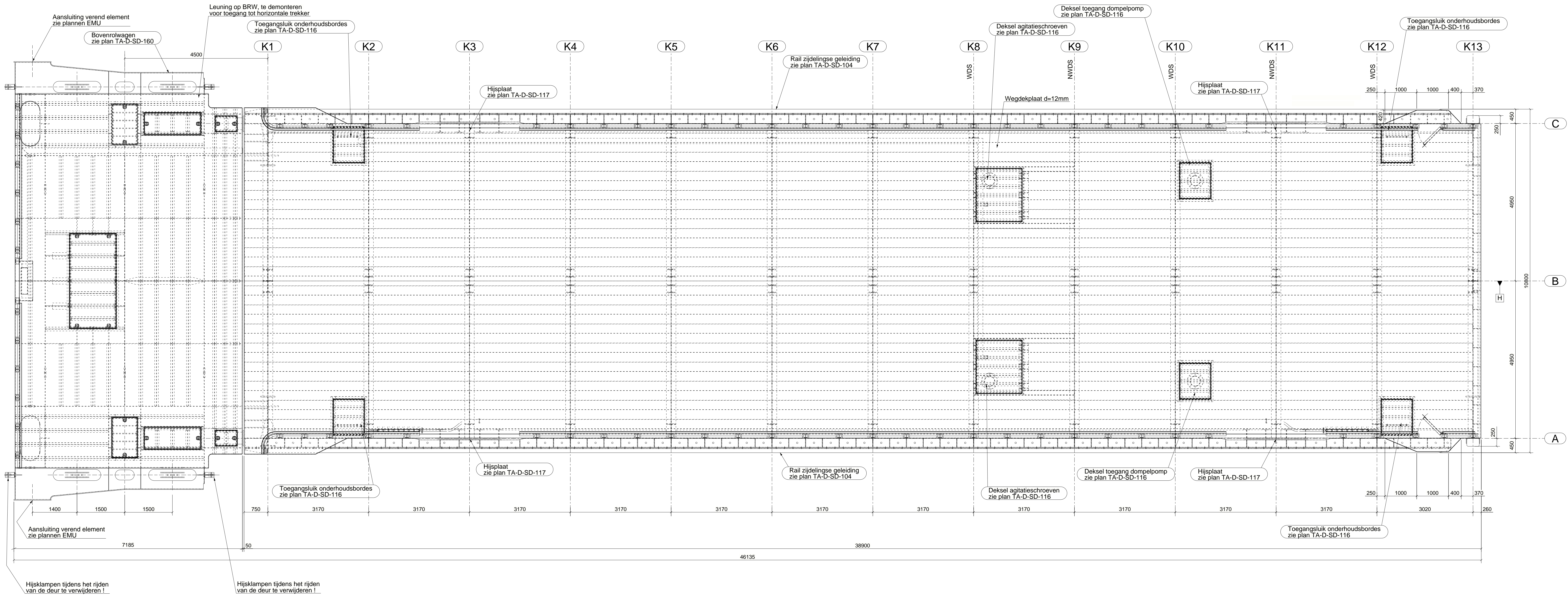
Bovenaanzicht Schaal: 1:50
