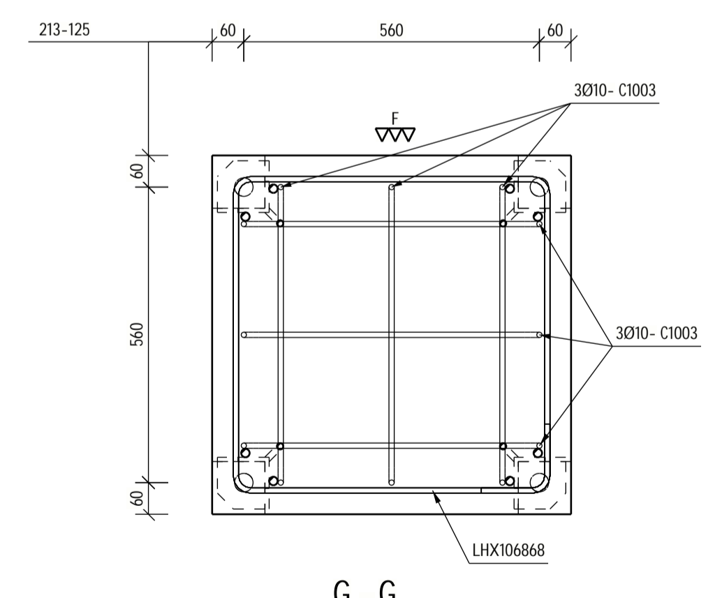
G-G 1:10
