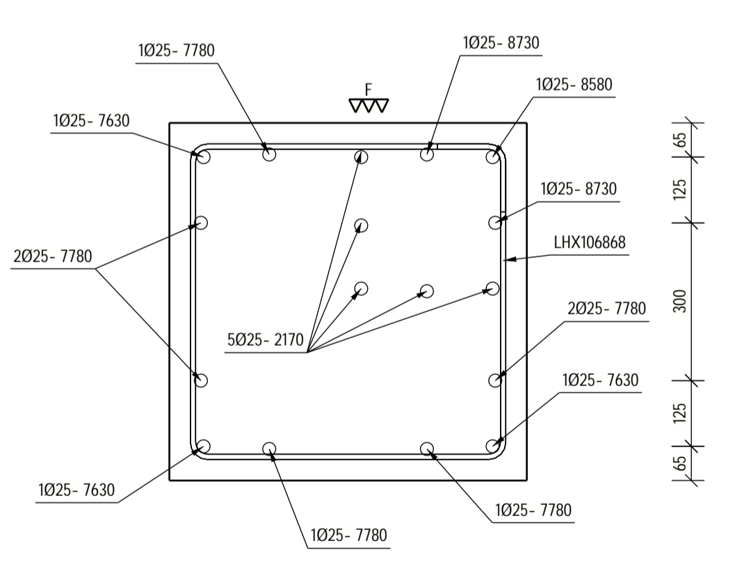
E-E 1:10
