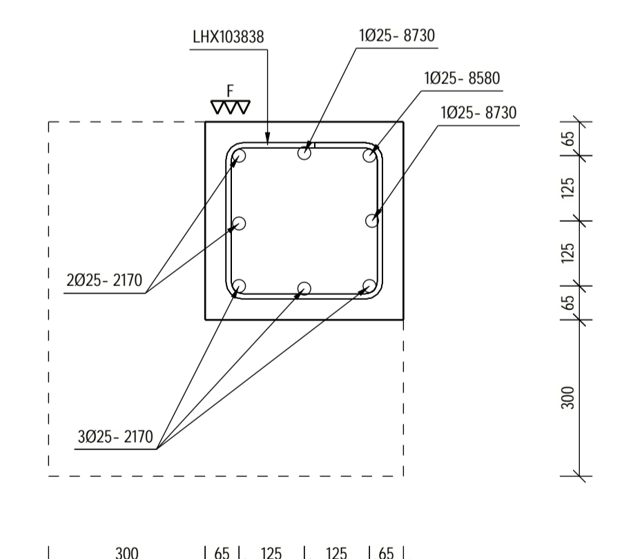
C-C 1:10
