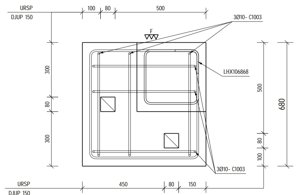
D-D 1:10
