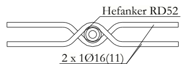
Wapening hefanker
