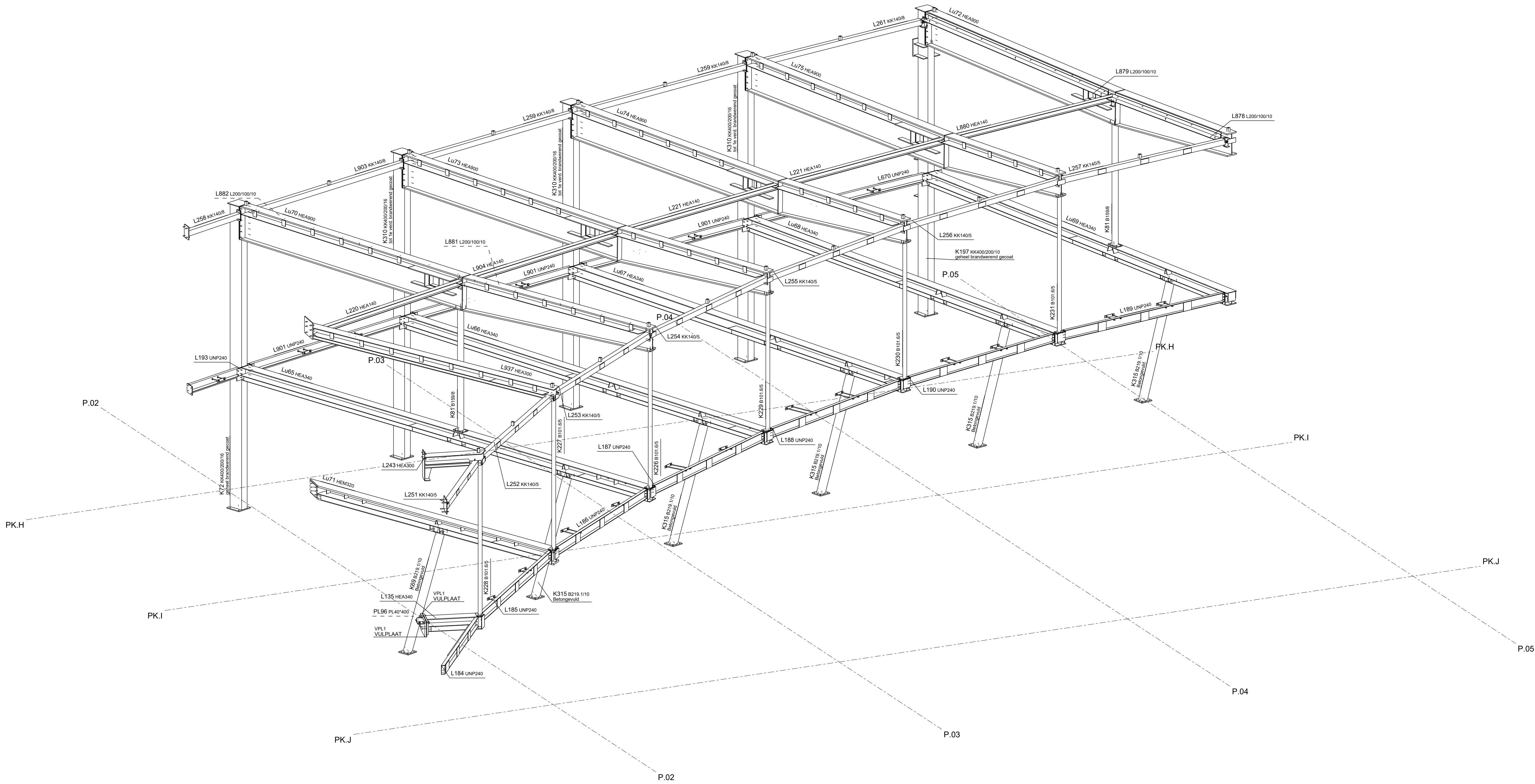
3d Tak Rechts, 1:50
