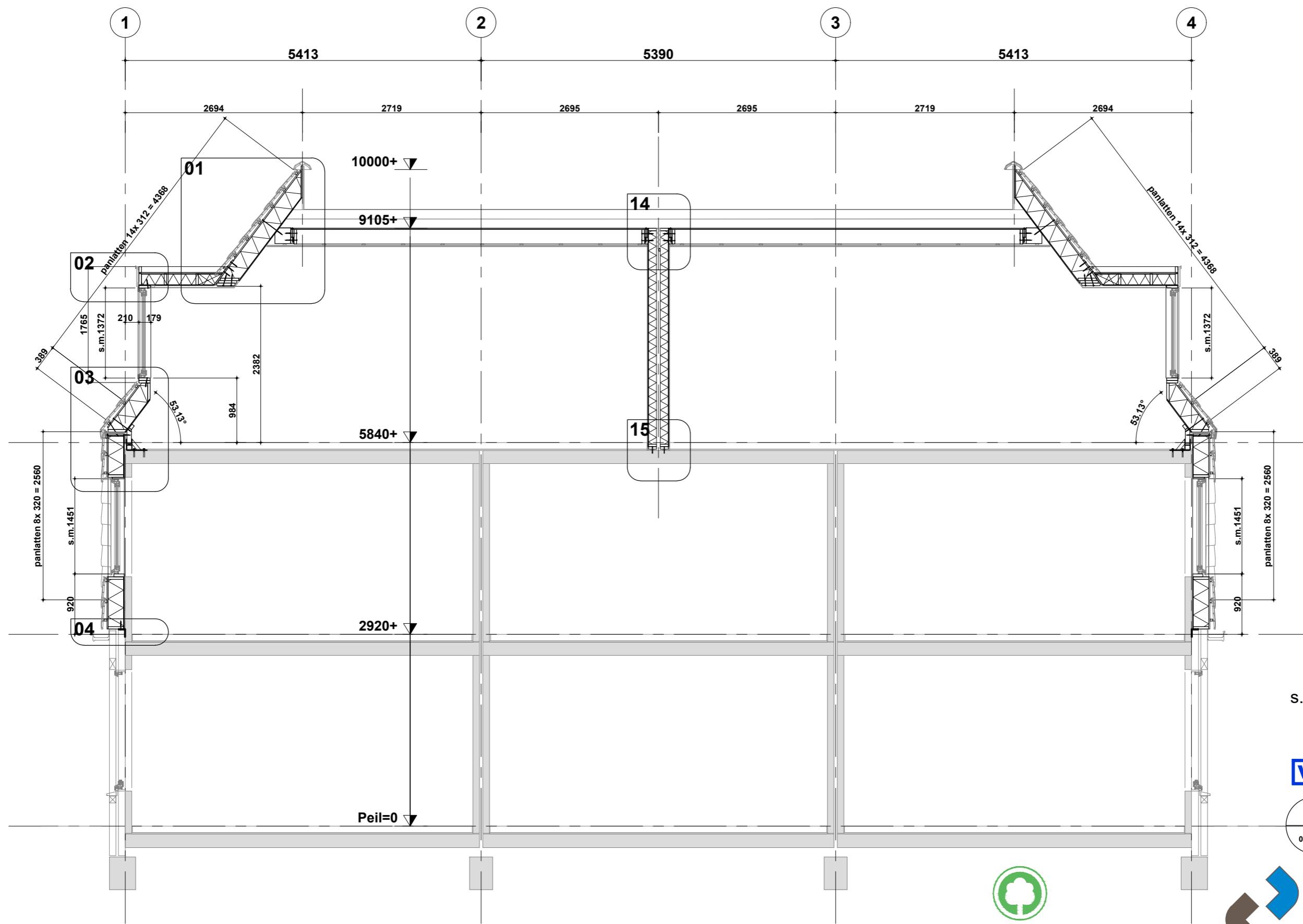
Doorsnede A-A
