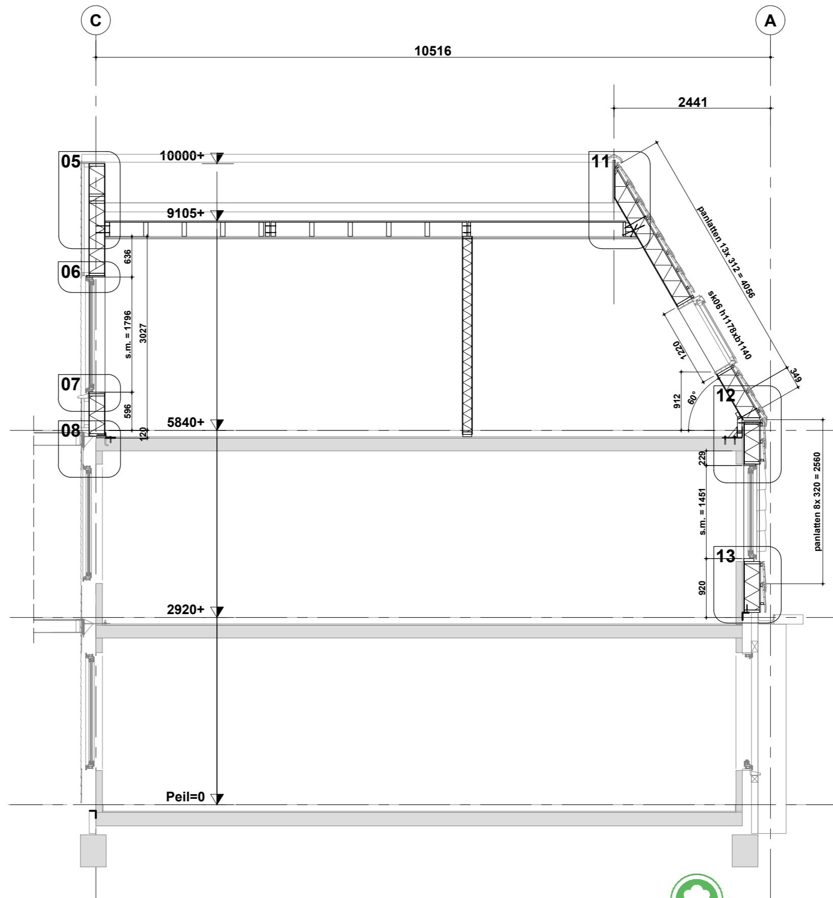
Doorsnede B-B
