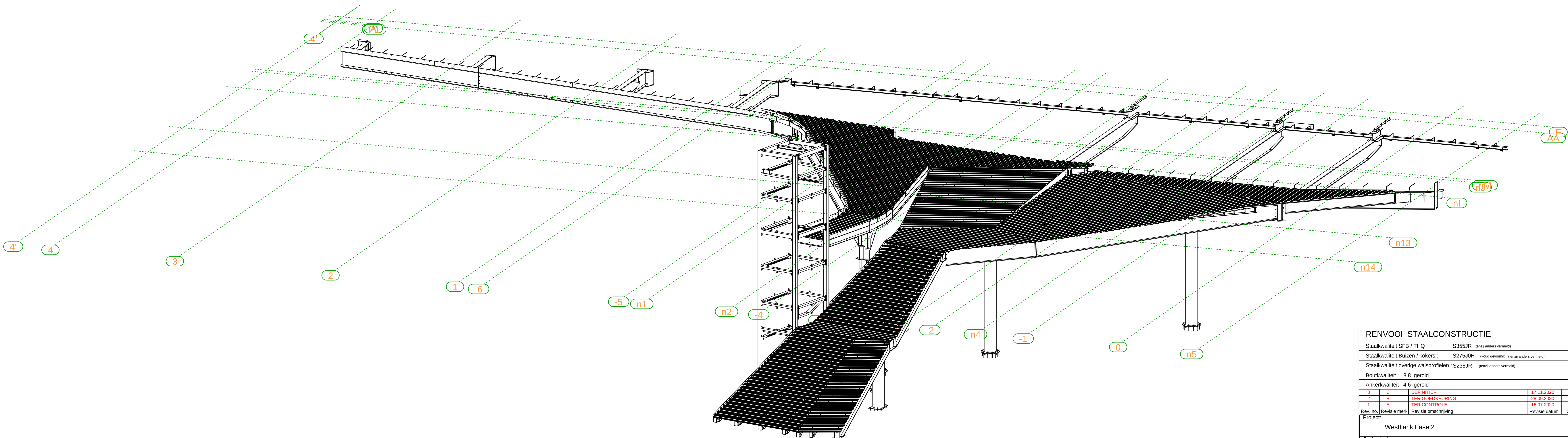
3D AANZICHT STAALCONSTRUCTIE WTC TRAP INCL. COMFLOR 1:75
