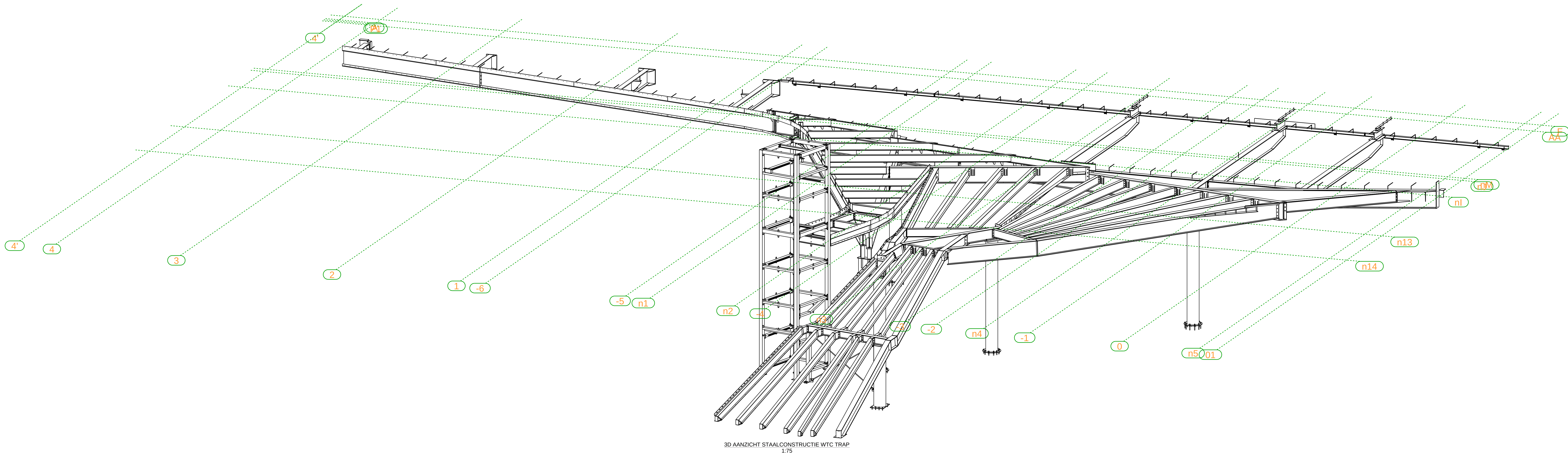
3D AANZICHT STAALCONSTRUCTIE WTC TRAP 1:75
