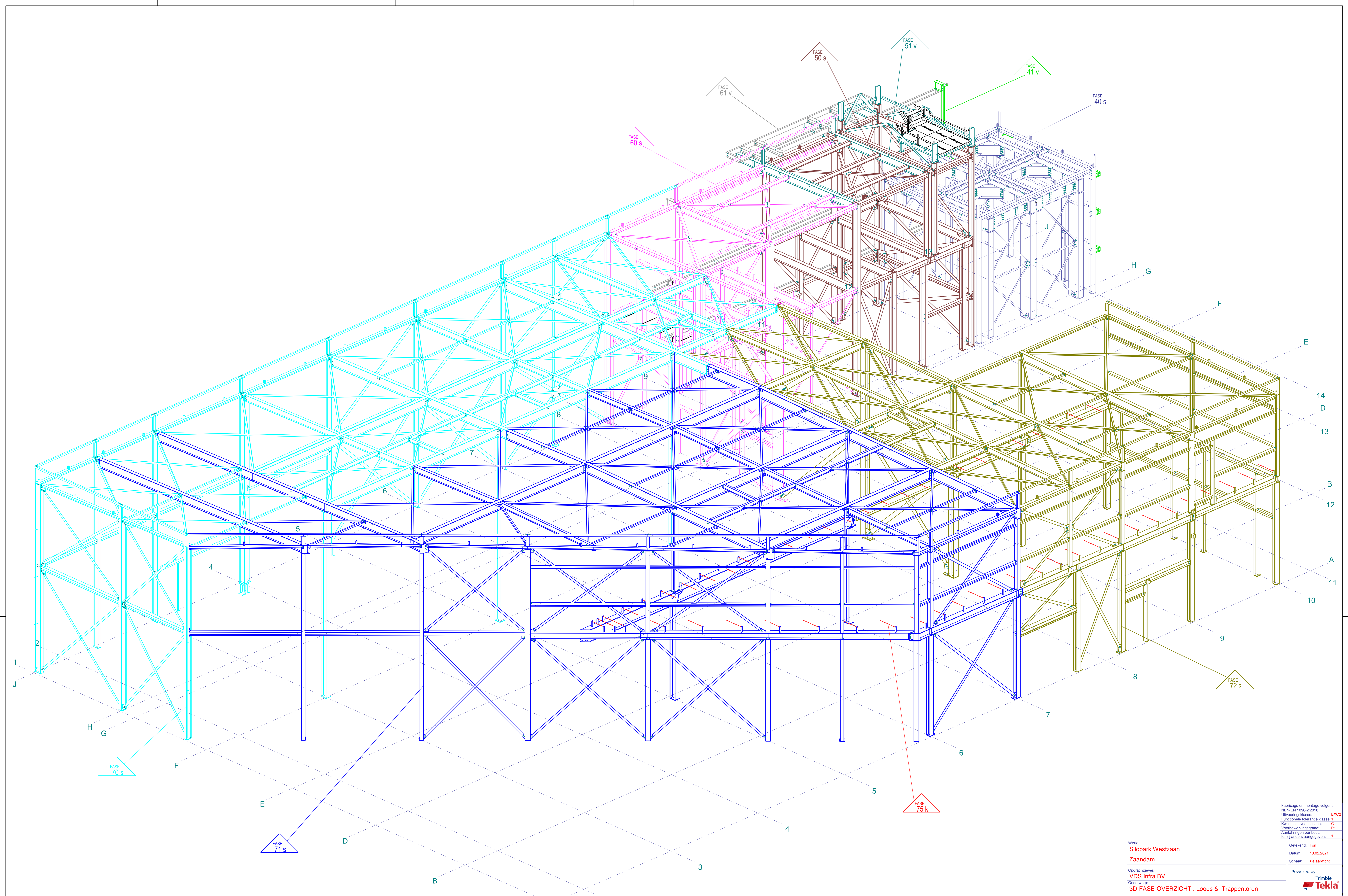
3D - FASE - OVERZICHT : LOODS & TRAPPENTOREN 1:50
