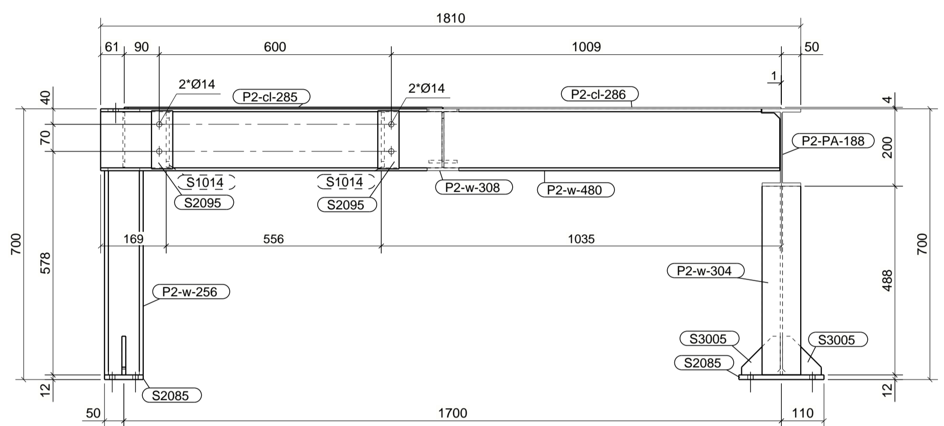
Sección D - D 1:10
