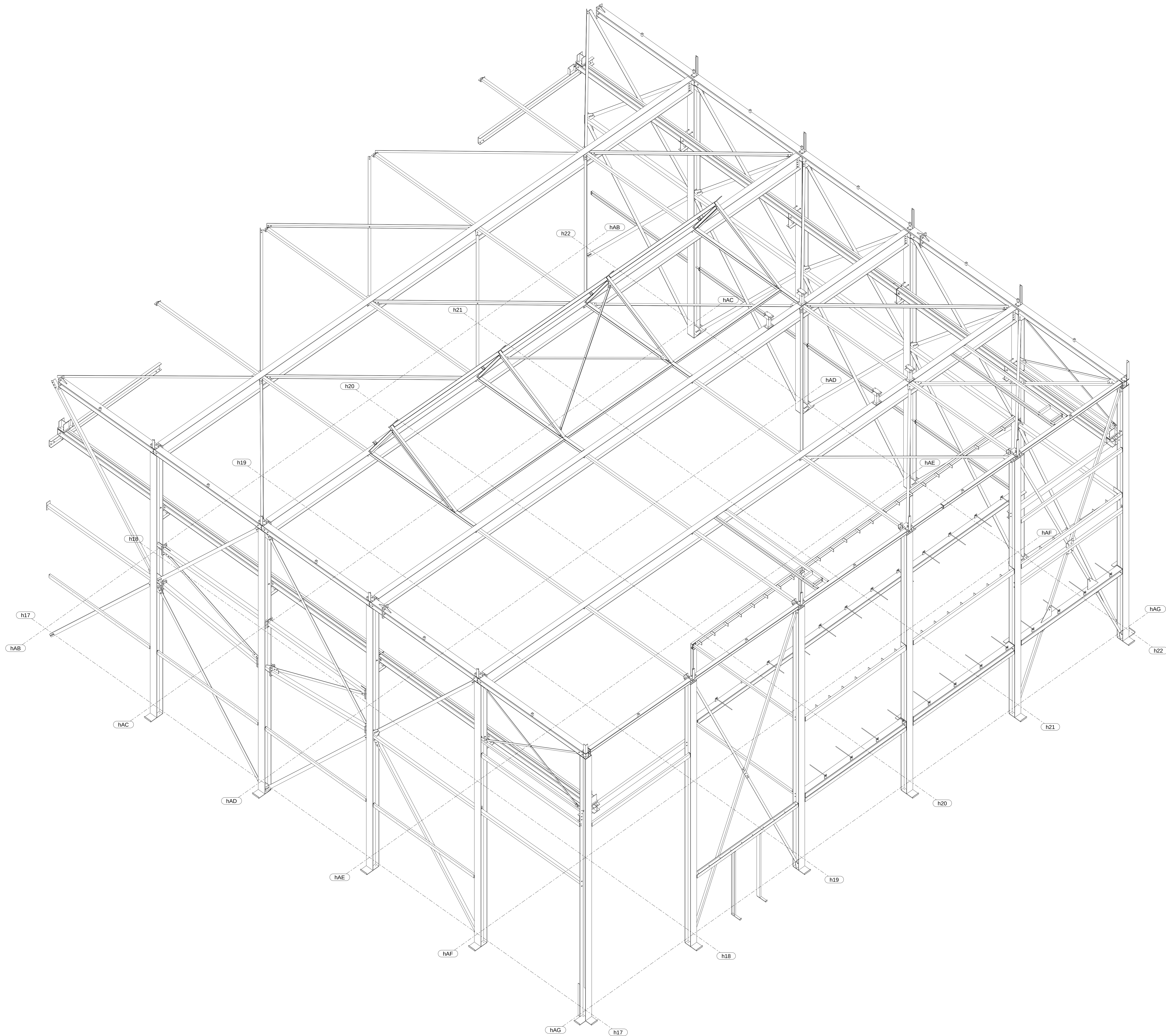
3D-OVERZICHT HAL 1 (BALANCING)
