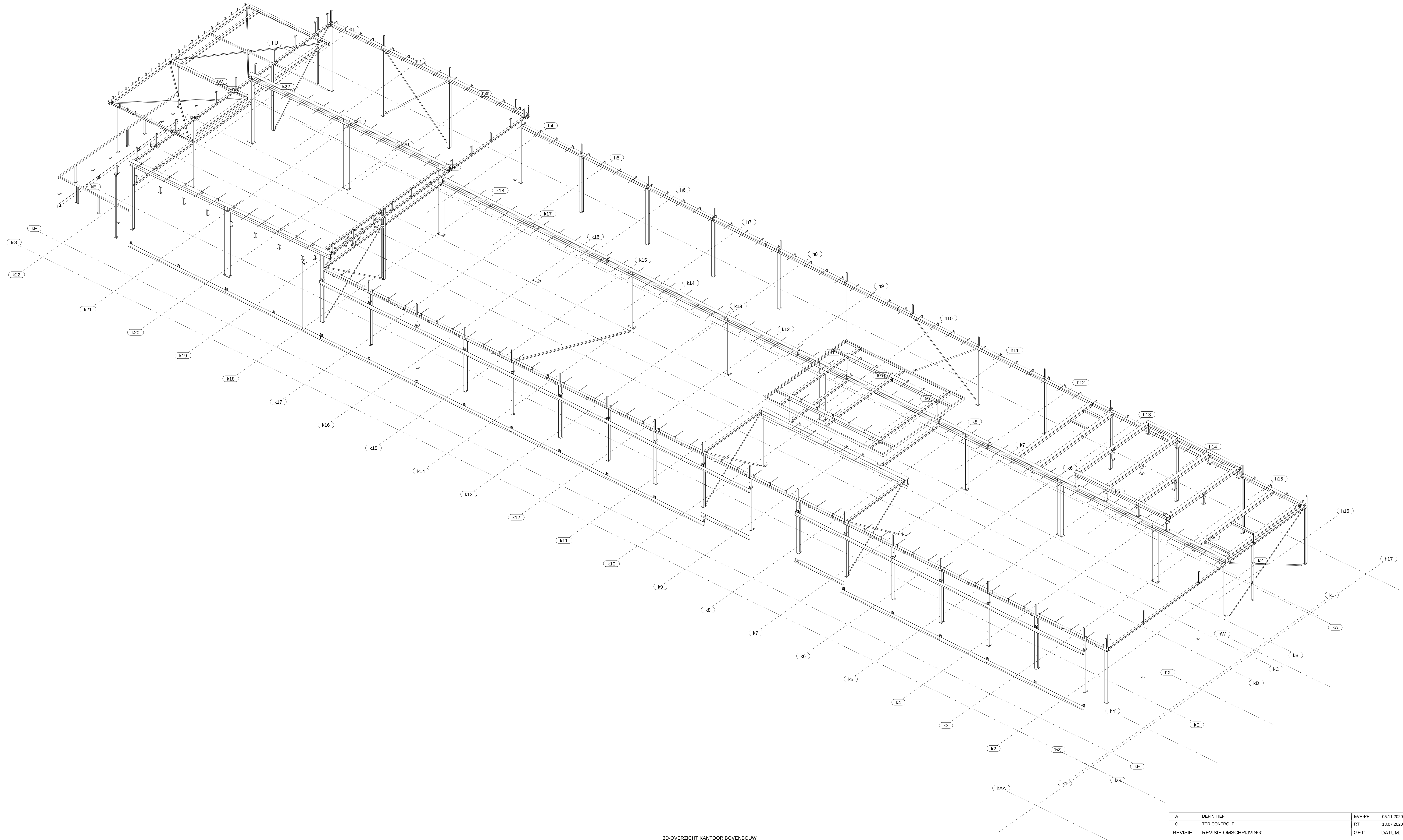
3D-OVERZICHT KANTOOR BOVENBOUW
