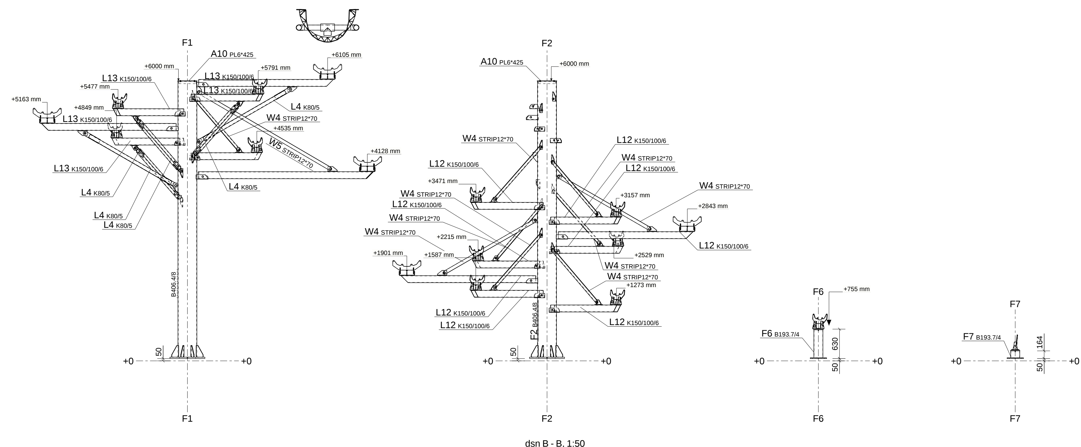
dsn B - B, 1:50
