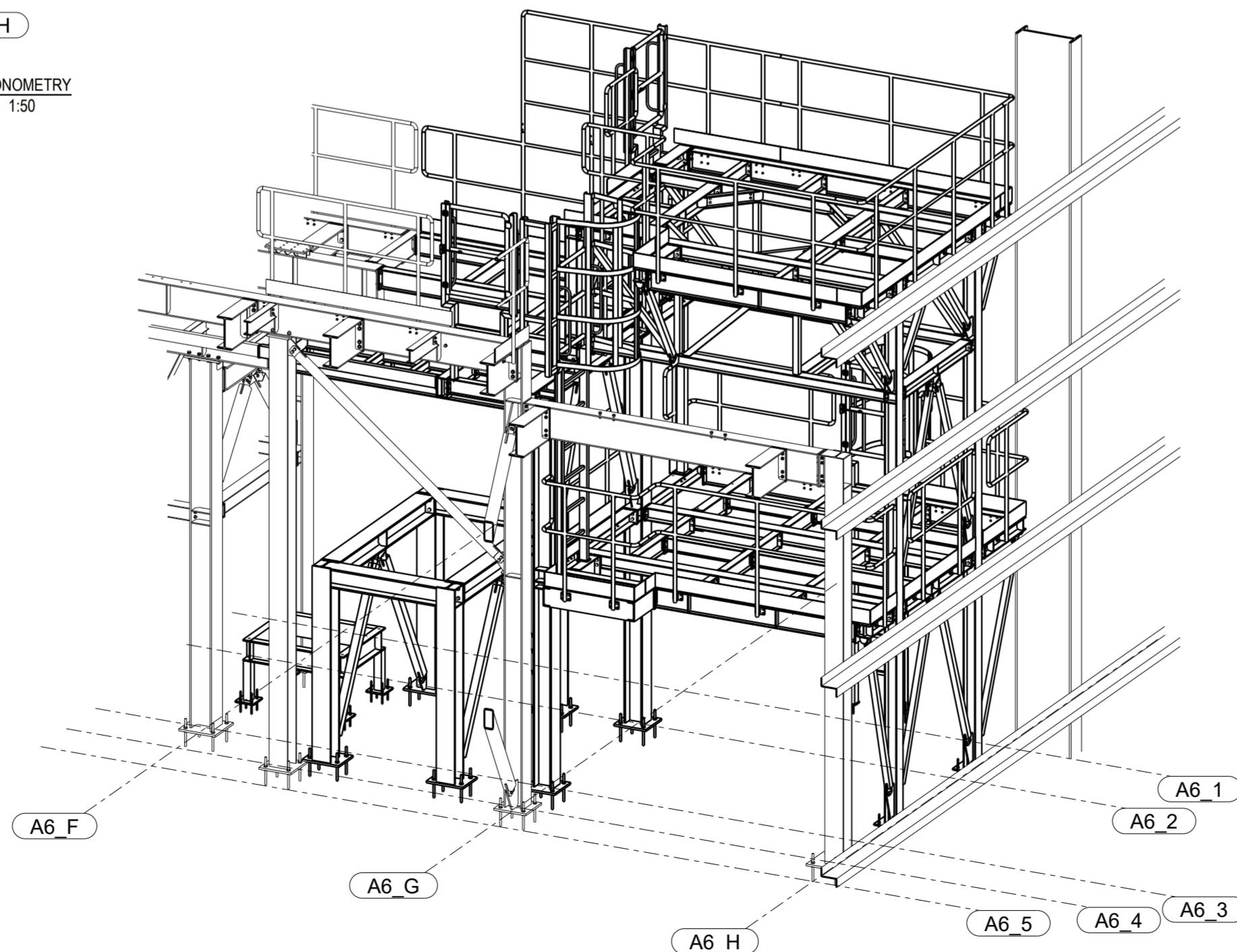
AXONOMETRY 1:50
