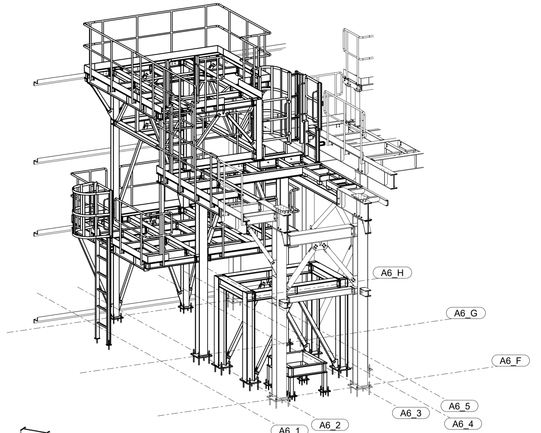
AXONOMETRY 1:50
