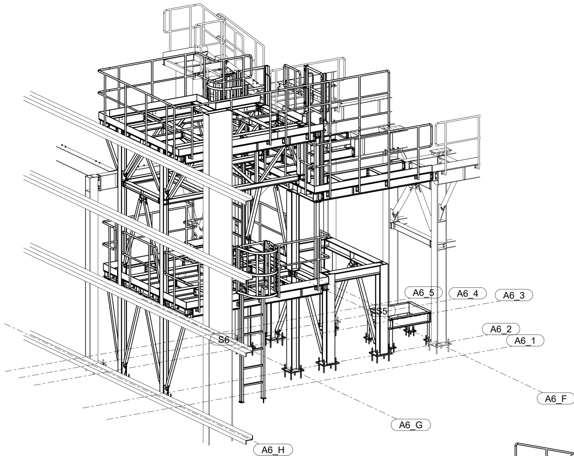
AXONOMETRY 1:50
