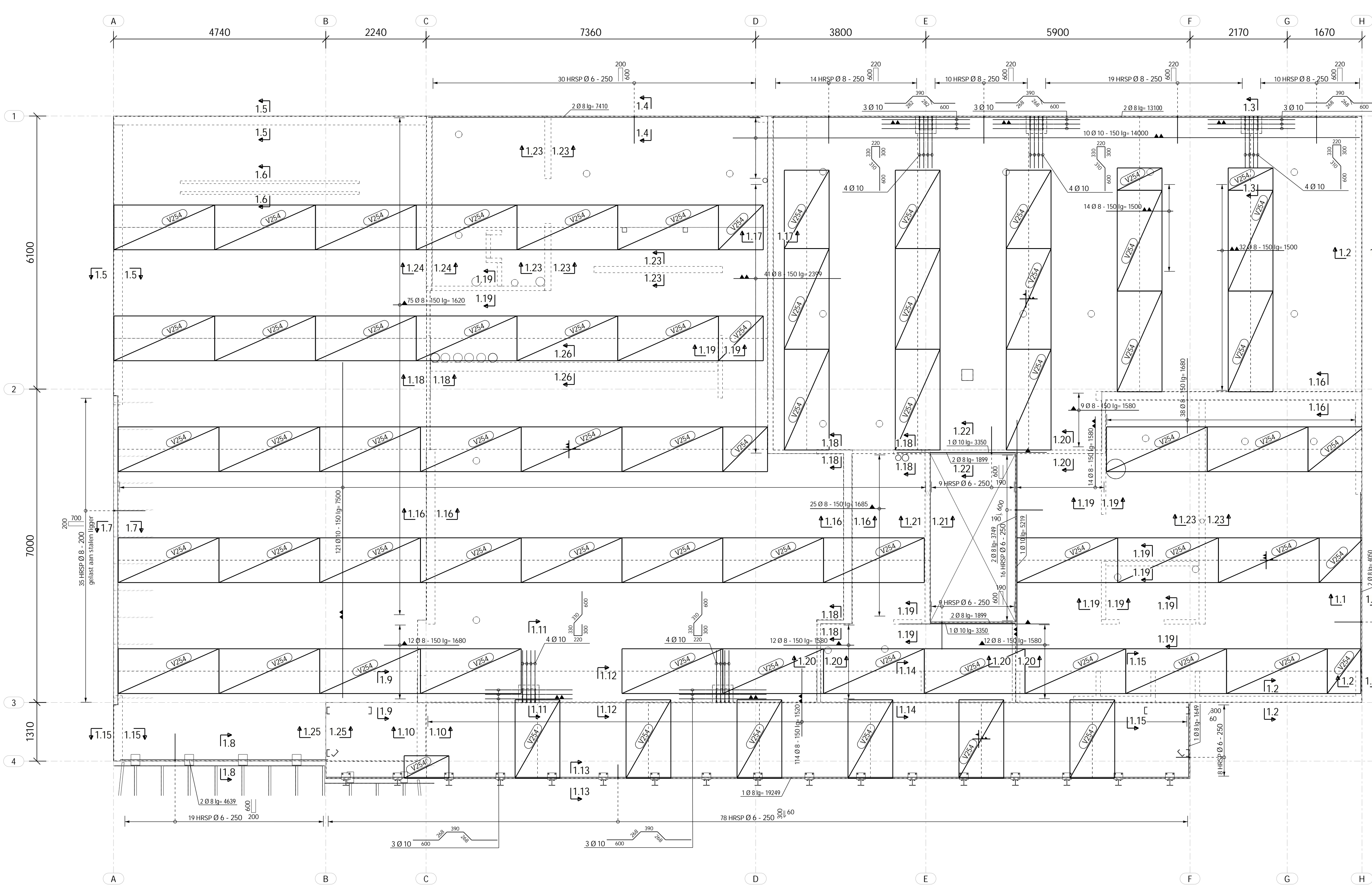
WAPENING OP DE PLAAT 1:50
