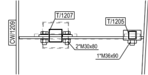
DETAIL B 1:15
