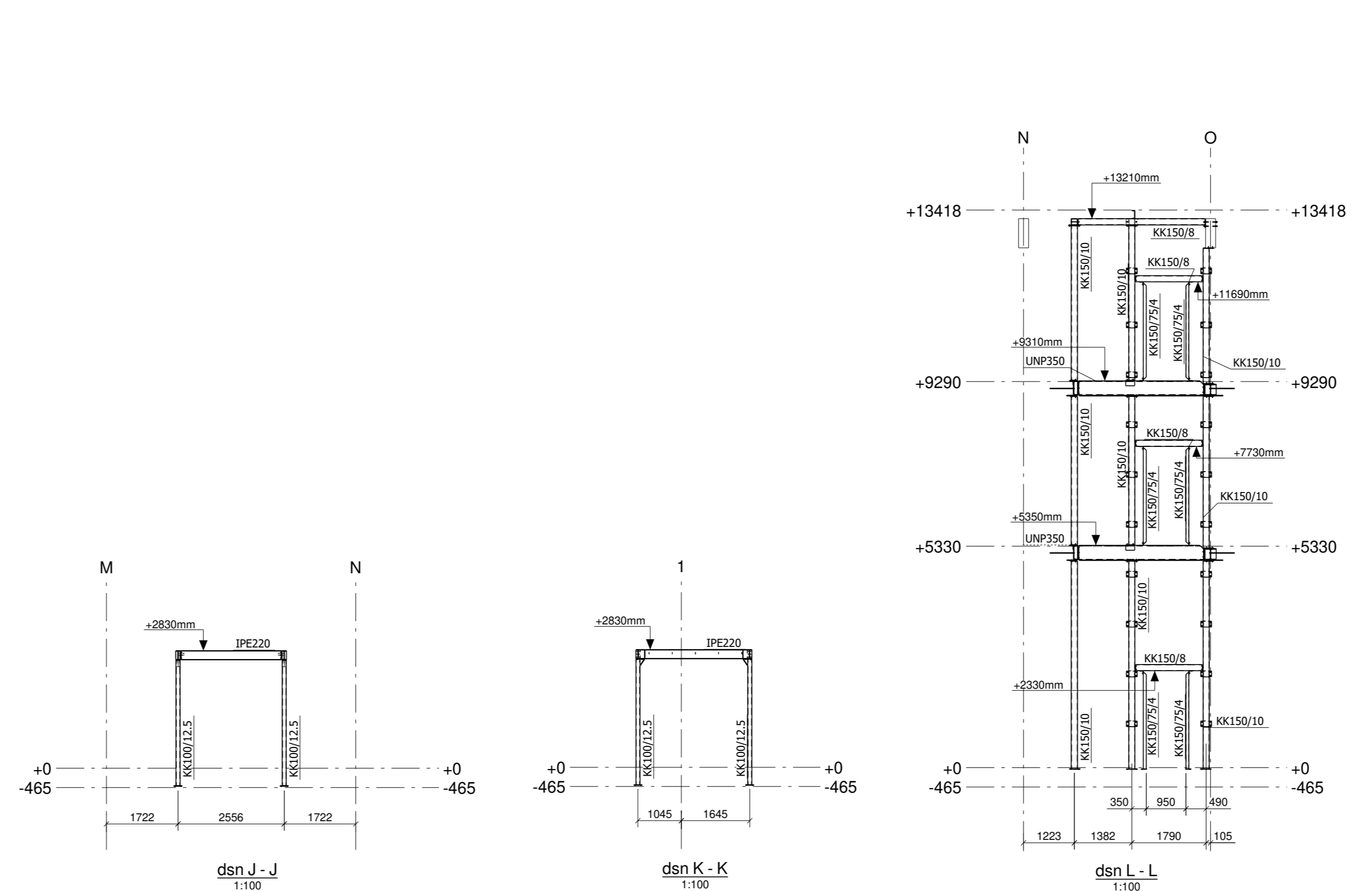
dsn J 1:100
