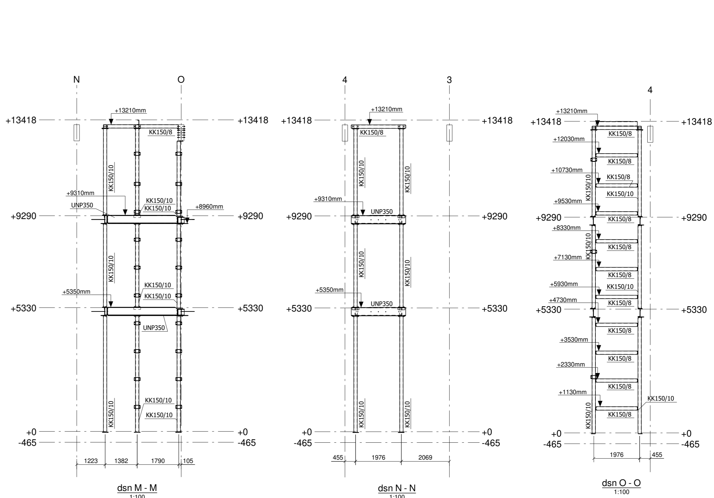
dsn M-M 1:100
