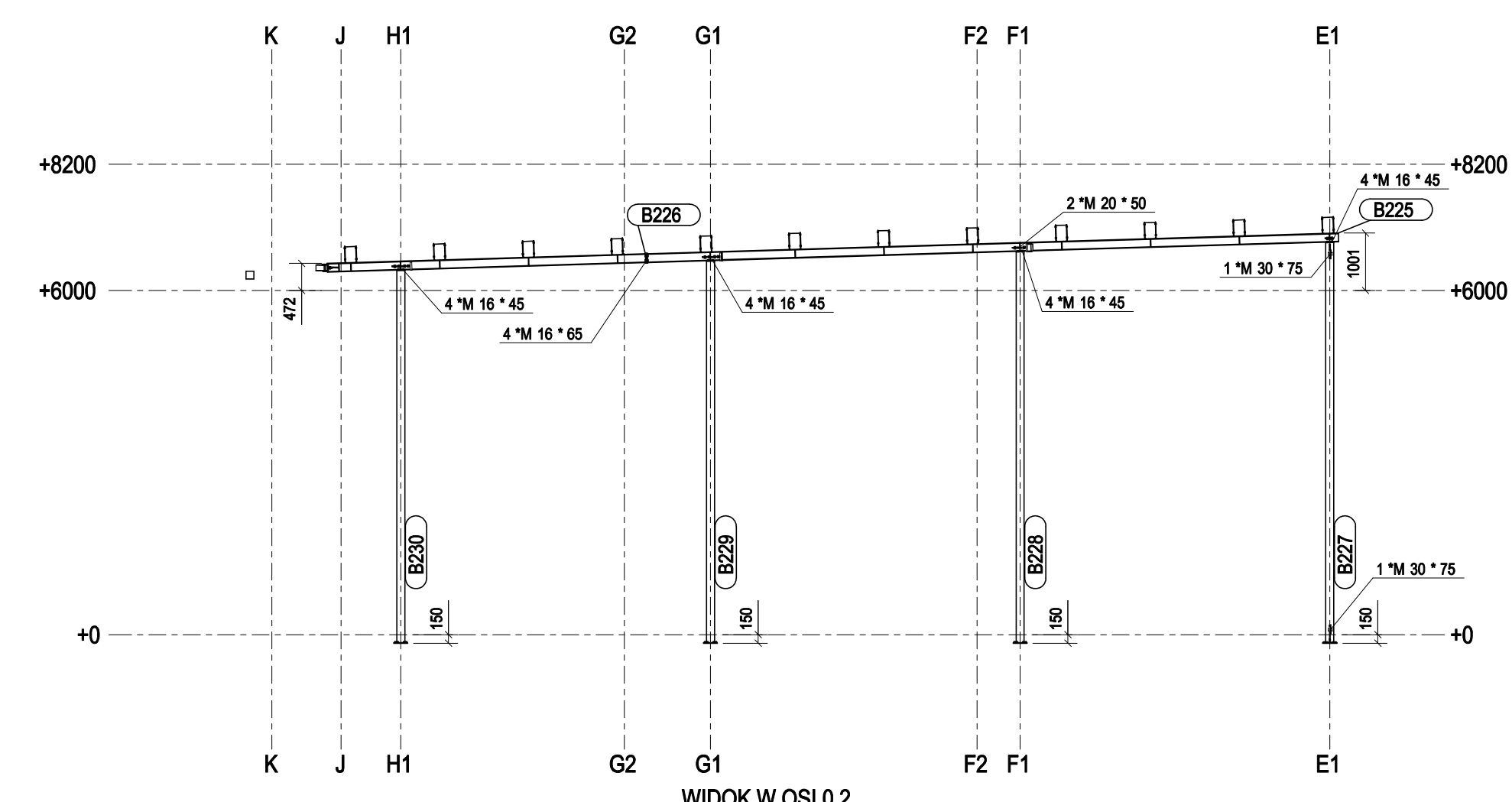
WIDOK W OSI 0.2 1:100
