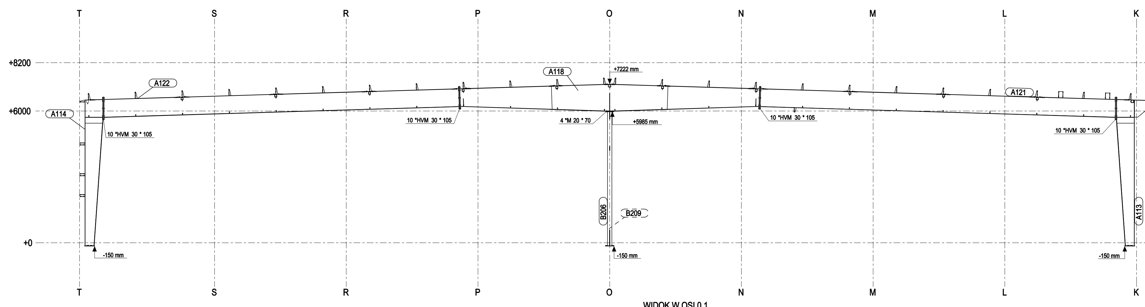
WIDOK W OSI 0.1 1:100
