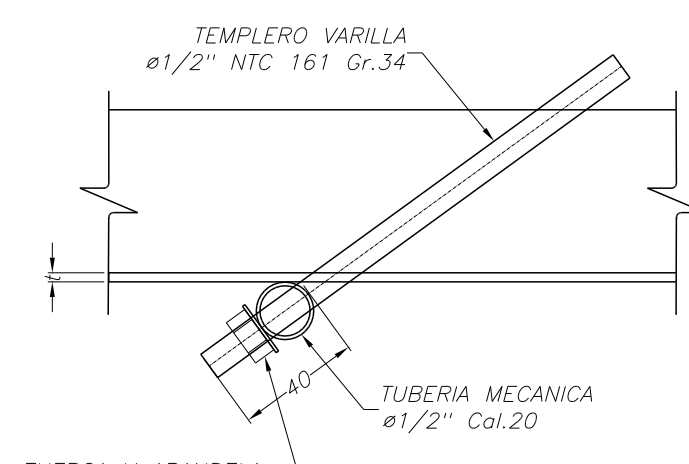
DETALLE TÍPICO TEMPLERO VARILLA 1:25
