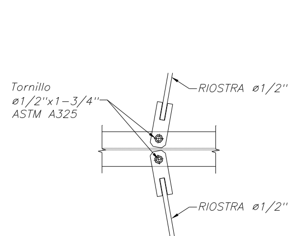
DETALLE TÍPICO RIOSTRA VARILLA 1:10
