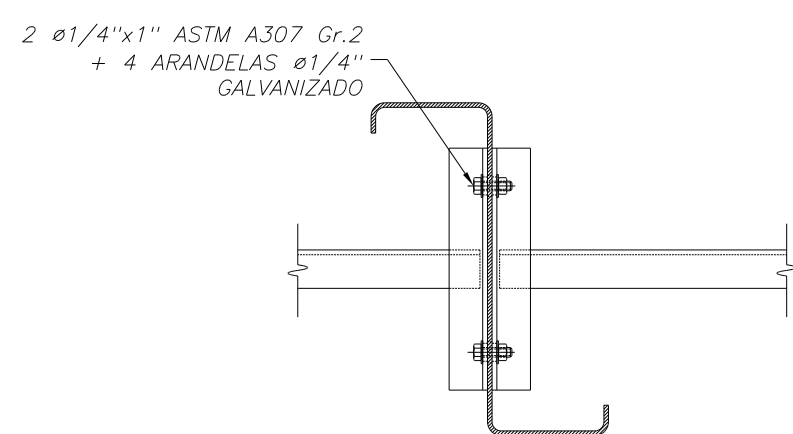
DETALLE TEMPLERO ANGULO EN CORREA "Z" INTERMEDIA
