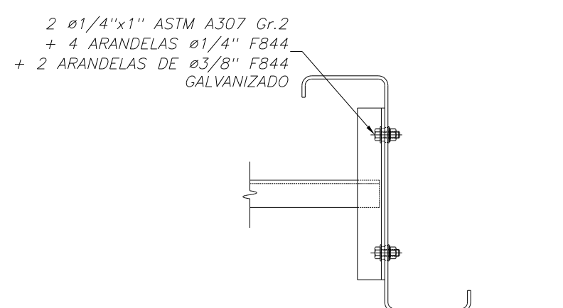
DETALLE TEMPLERO ANGULO EN CORREA "Z" EXTREMA
