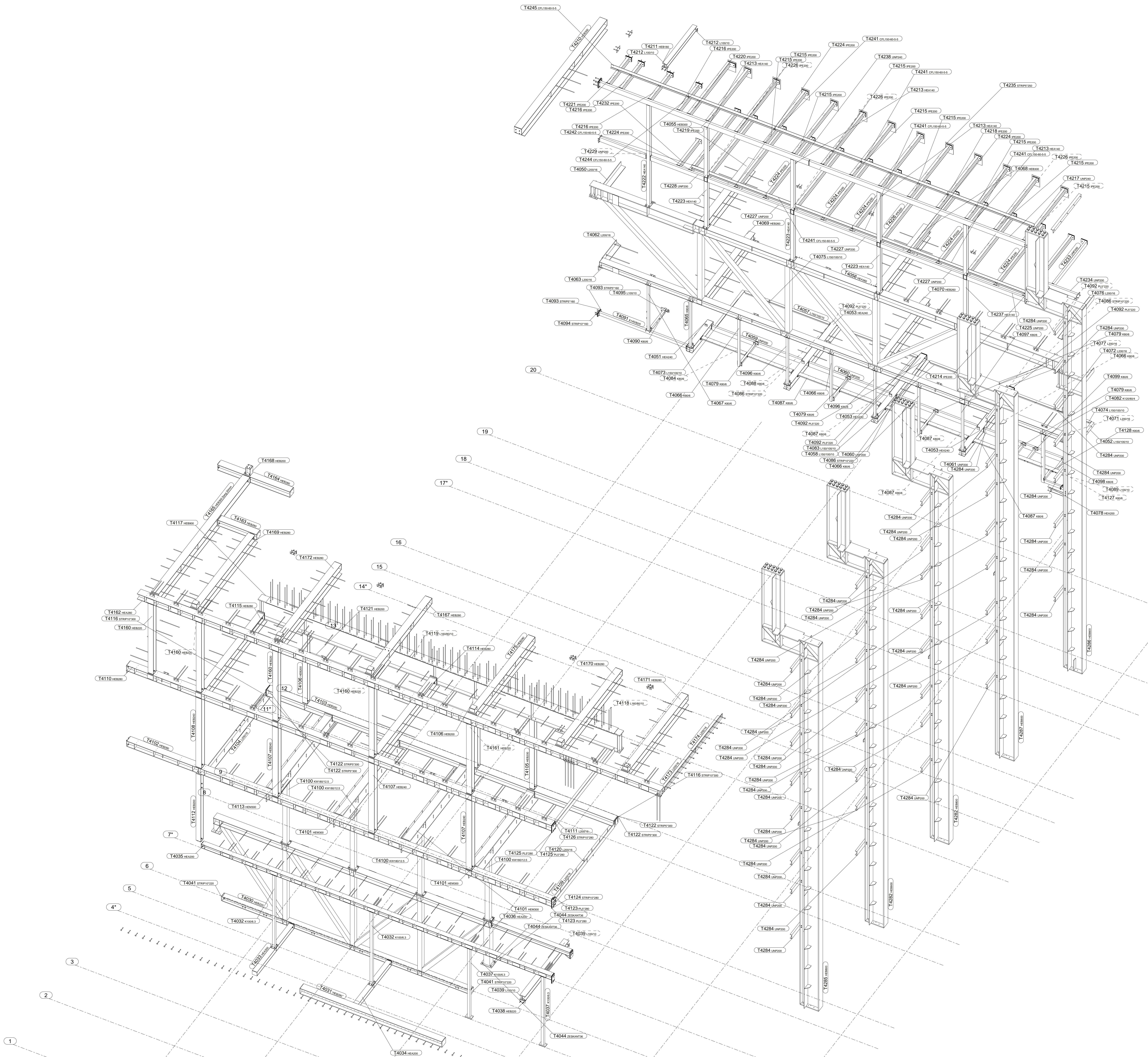
3D beganegrond t/m 5e verdieplingsvloer 1:50
