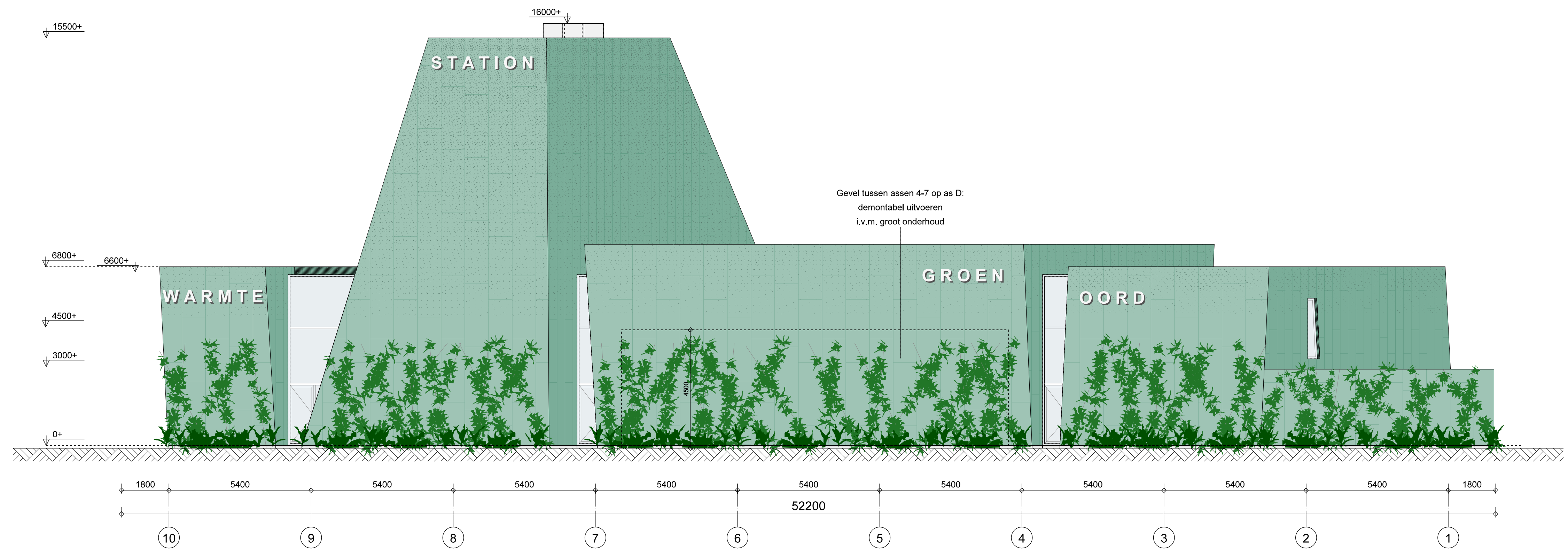
noordgevel
