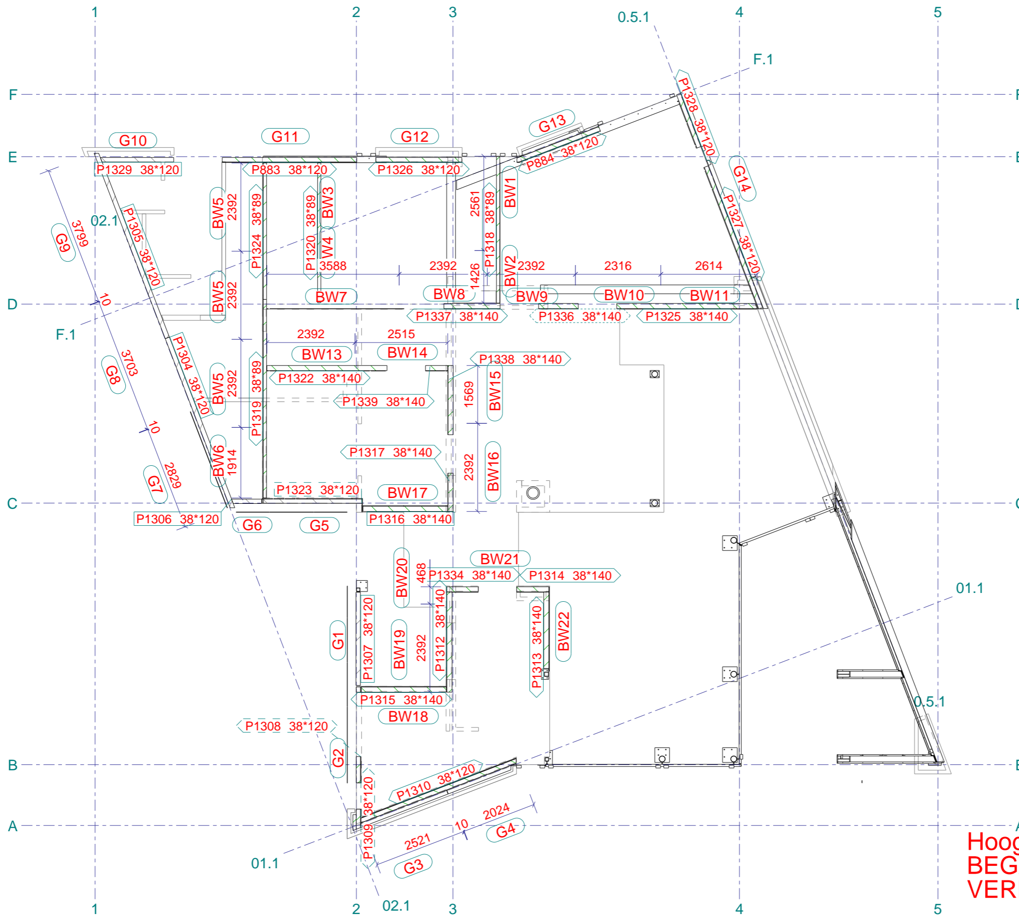
Bovenaanzicht BEG 1:100
