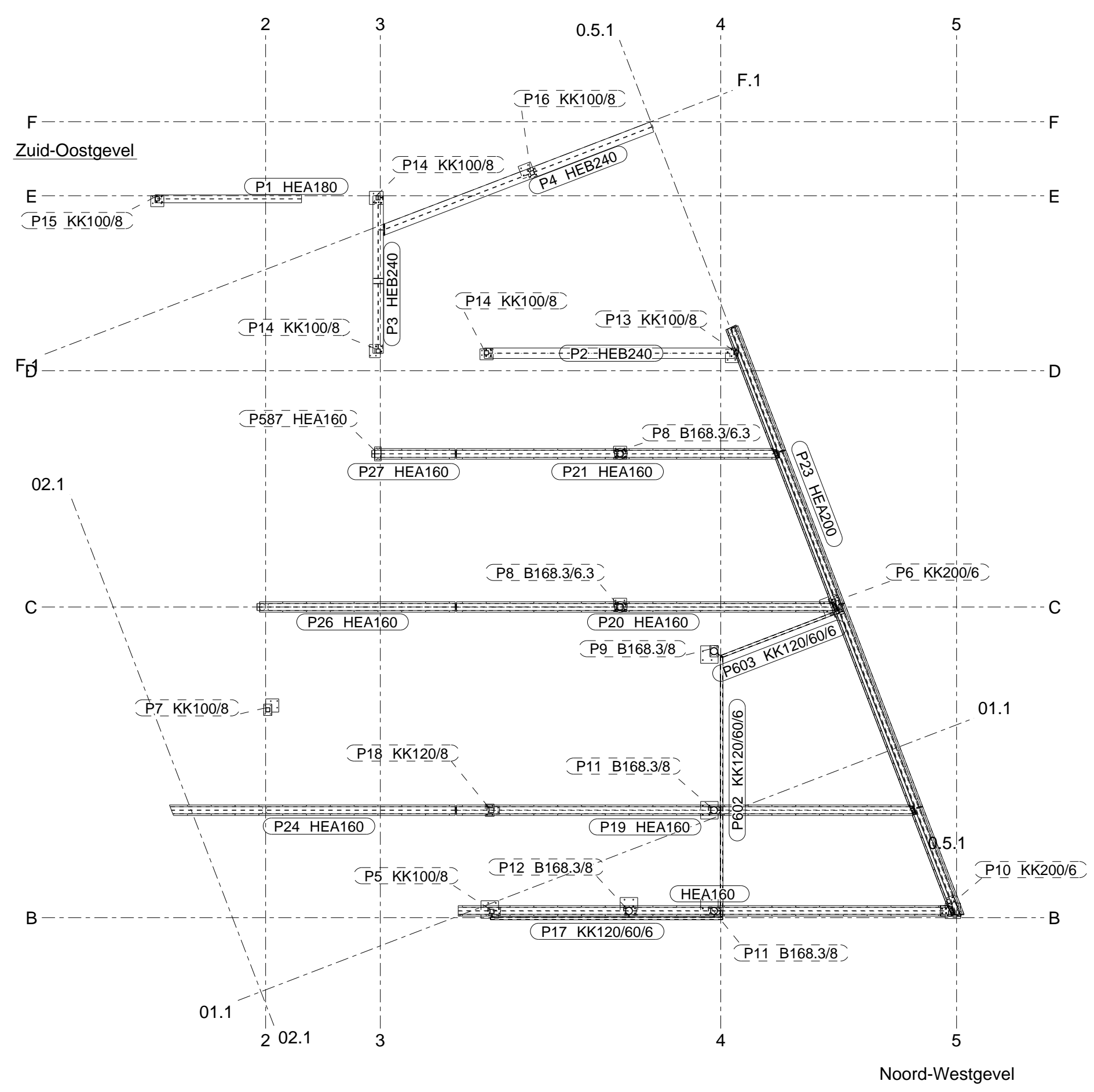
Plattegrond 1:100
