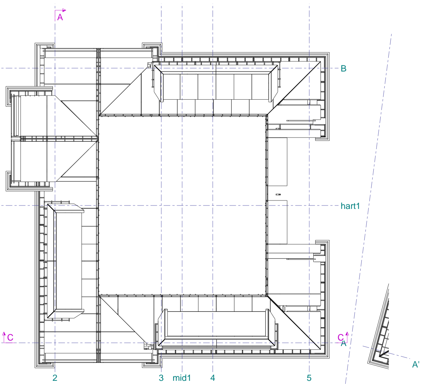
LEGPLAN 1:150
