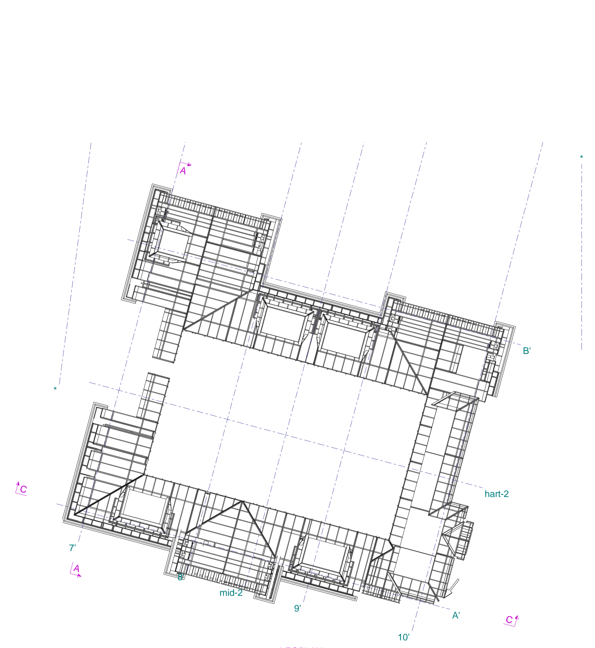
LEGPLAN 1:150
