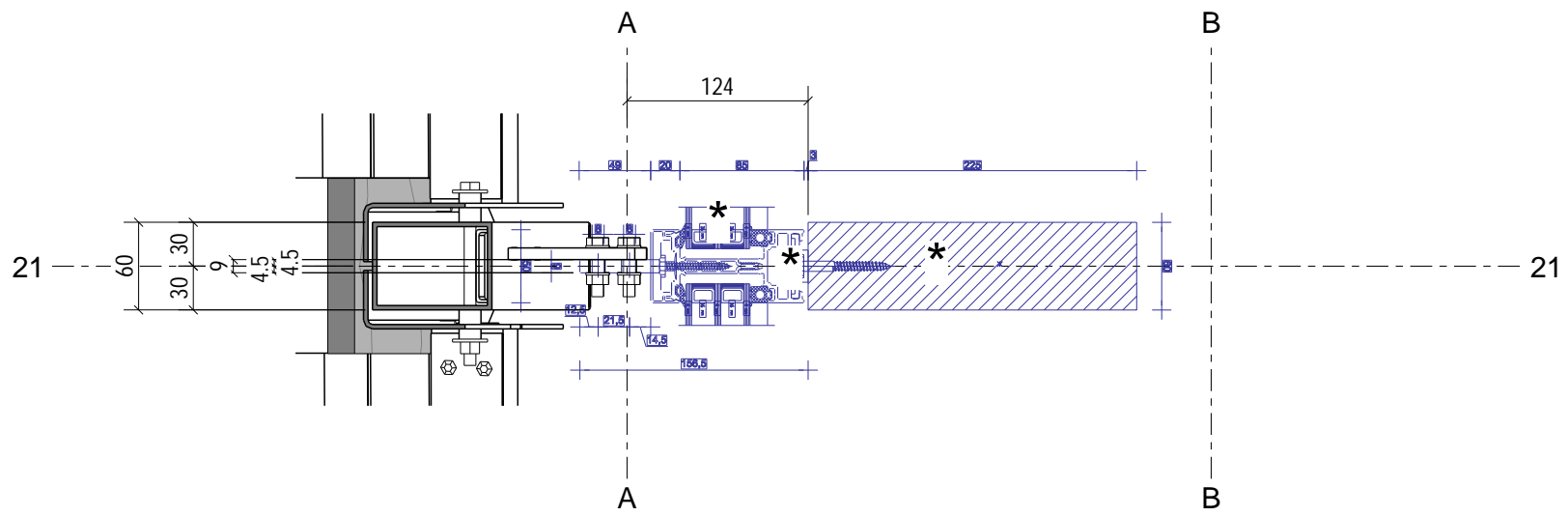
dsn A - A, 1:5
