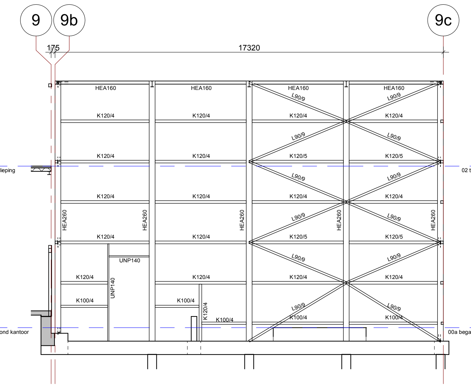
Aanzicht as-F7 1 : 100
