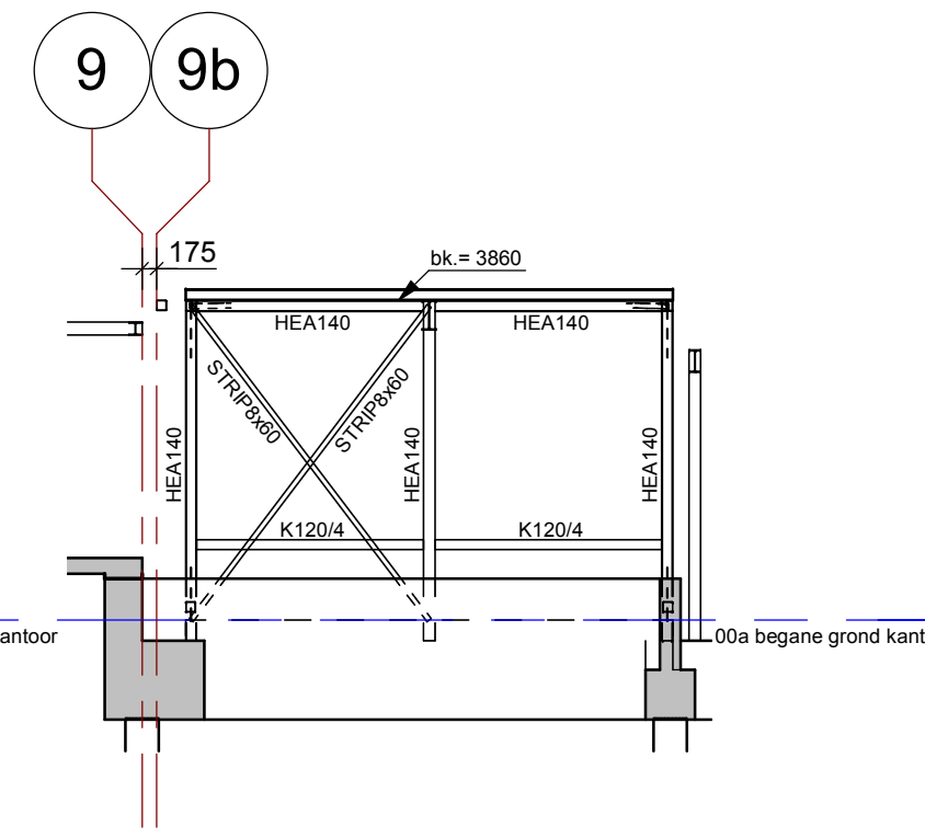
Aanzicht as-G' 1 : 100
