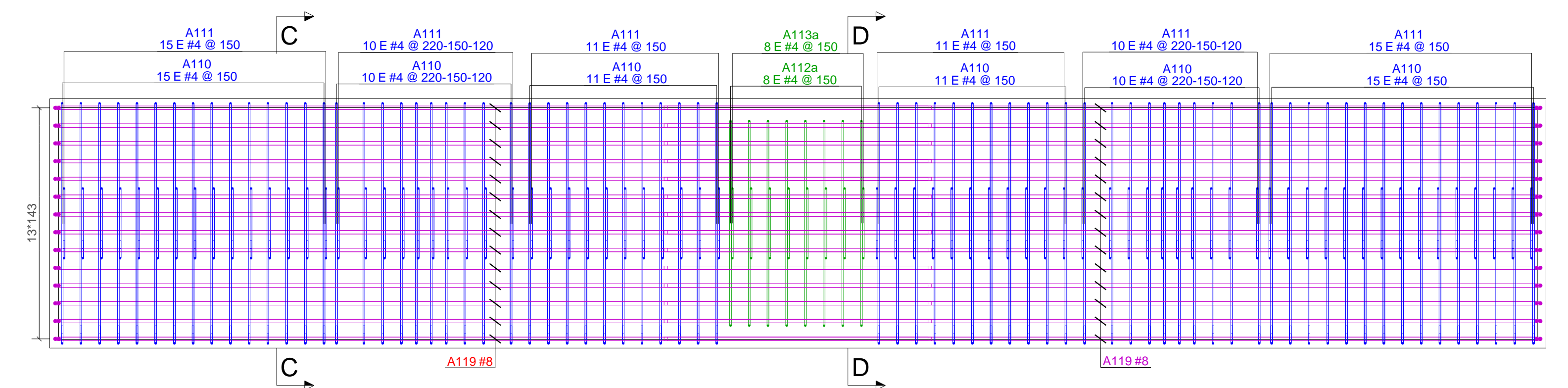
REFUERZO - VISTA SUPERIOR VIGA CAJÓN EJE 5 Esc: 1:30
