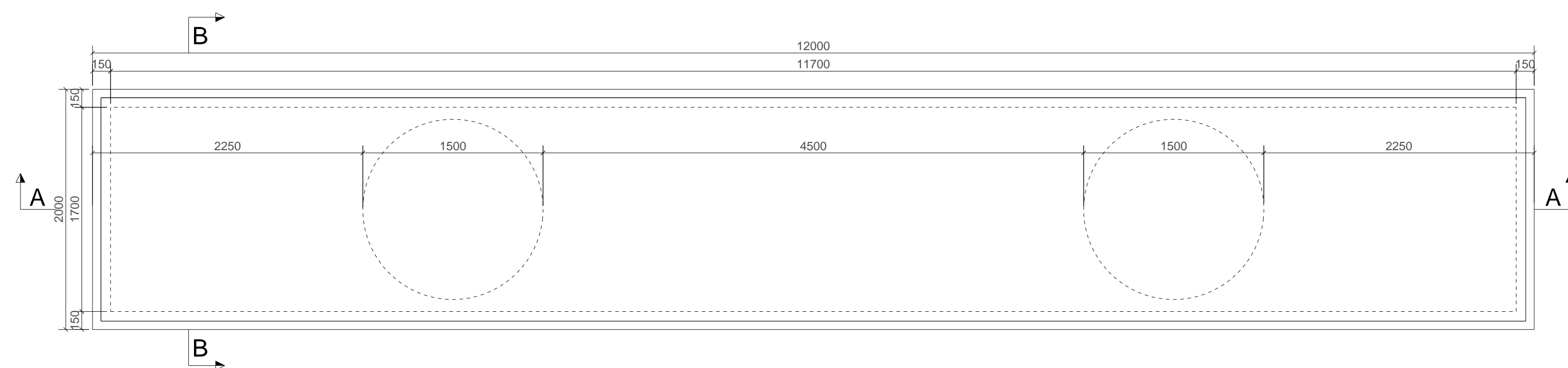
VISTA PLANTA - VIGA CAJÓN EJE 5 Esc: 1:30
