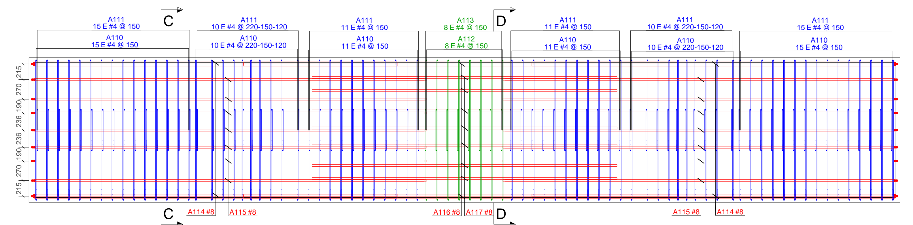
REFUERZO - VISTA INFERIOR VIGA CAJÓN EJE 5 Esc: 1:30
