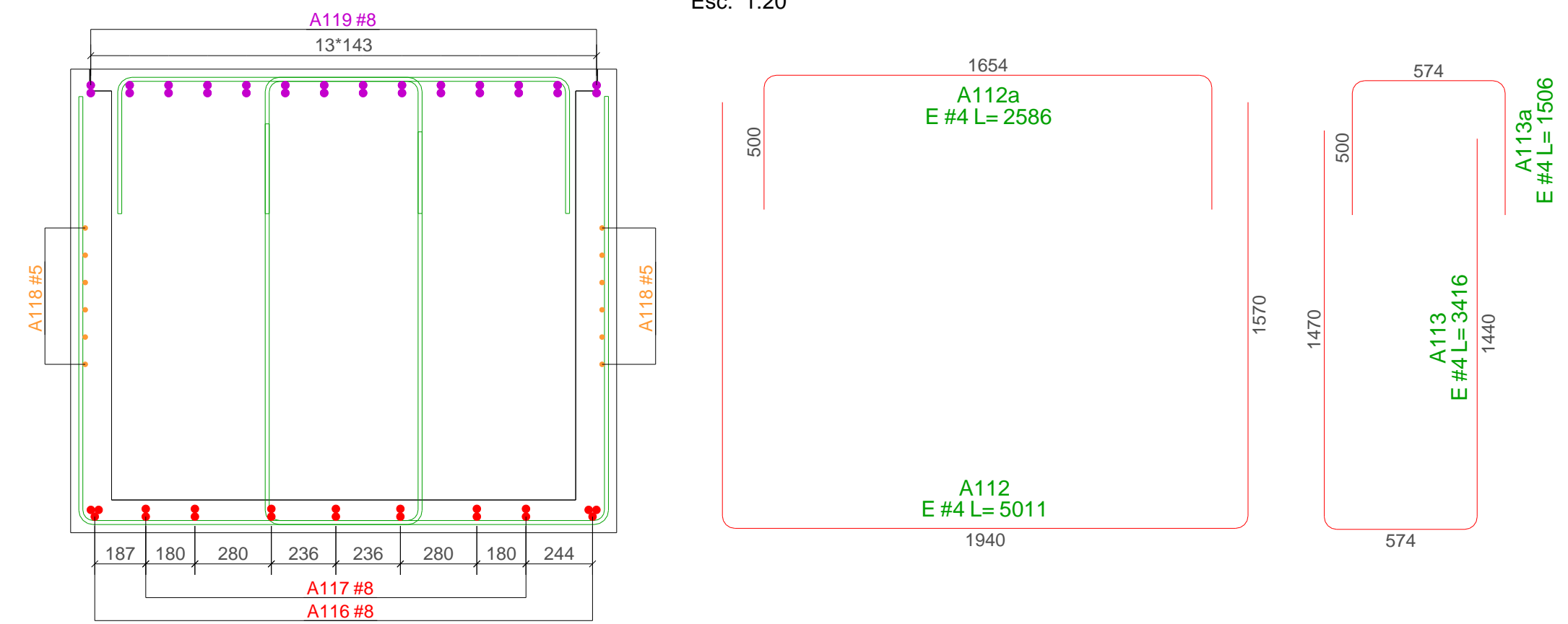
CORTE D - D Esc: 1:20
