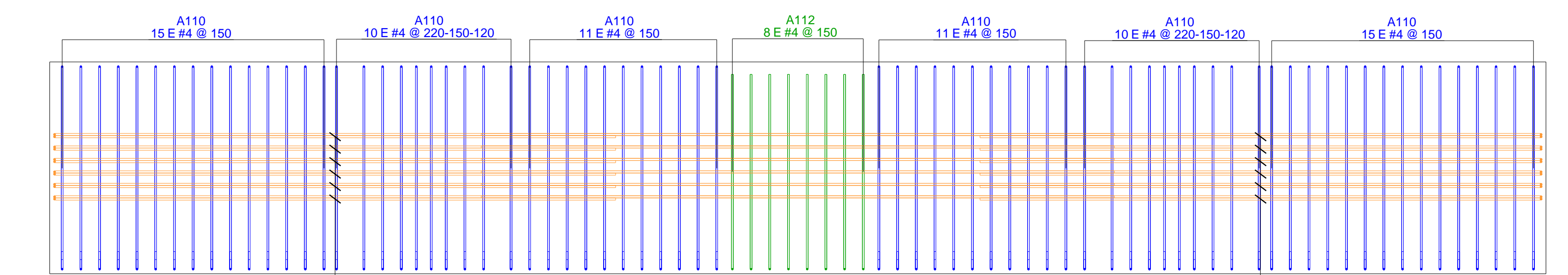
REFUERZO - VISTA LATERAL VIGA CAJÓN EJE 5 Esc: 1:30
