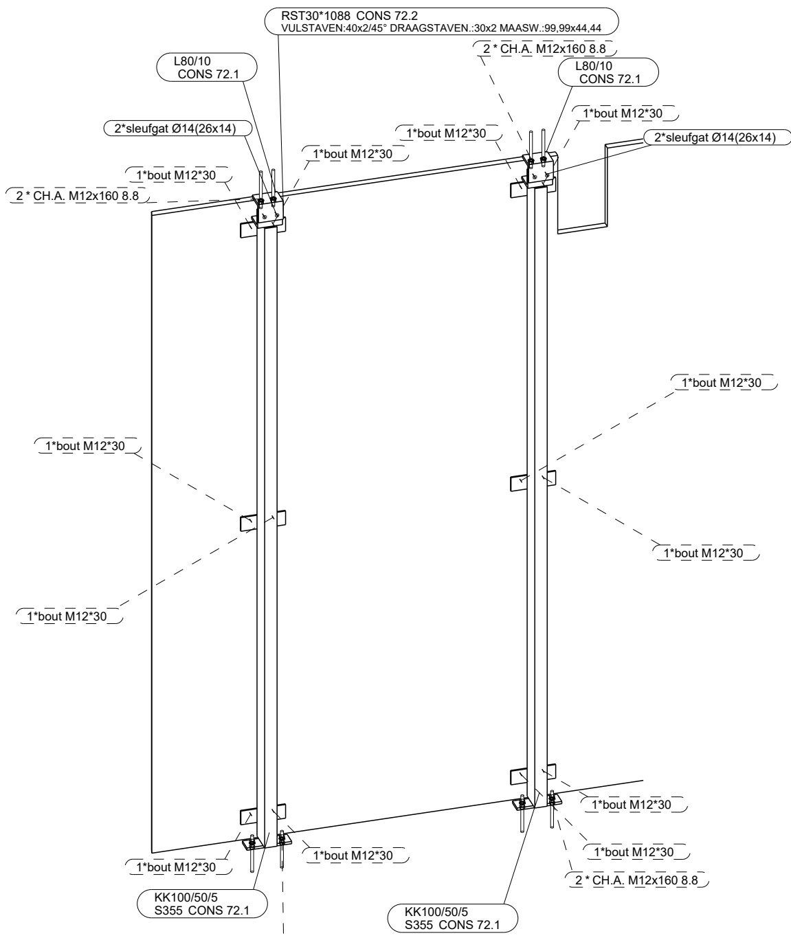
3D principe hekwerk (van binnenuit), 1:20
