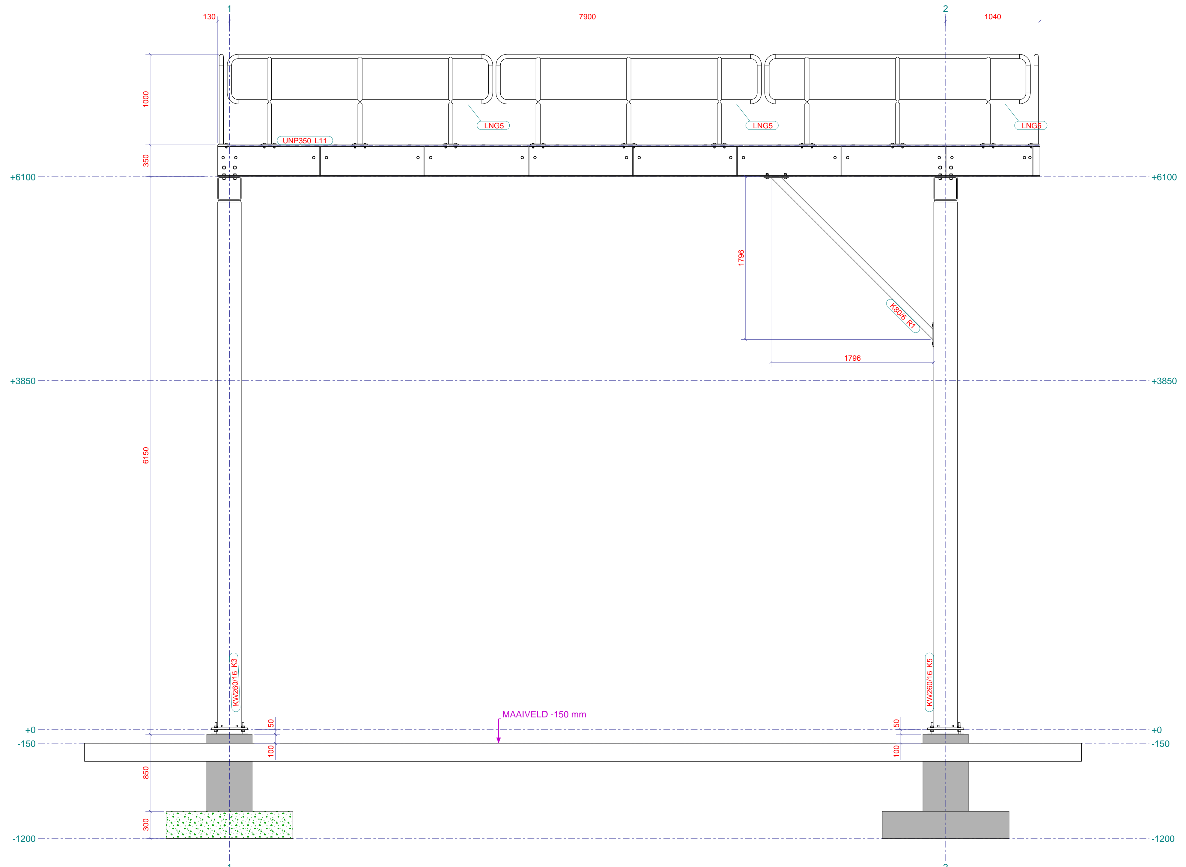
Vooraanzicht 1:25
