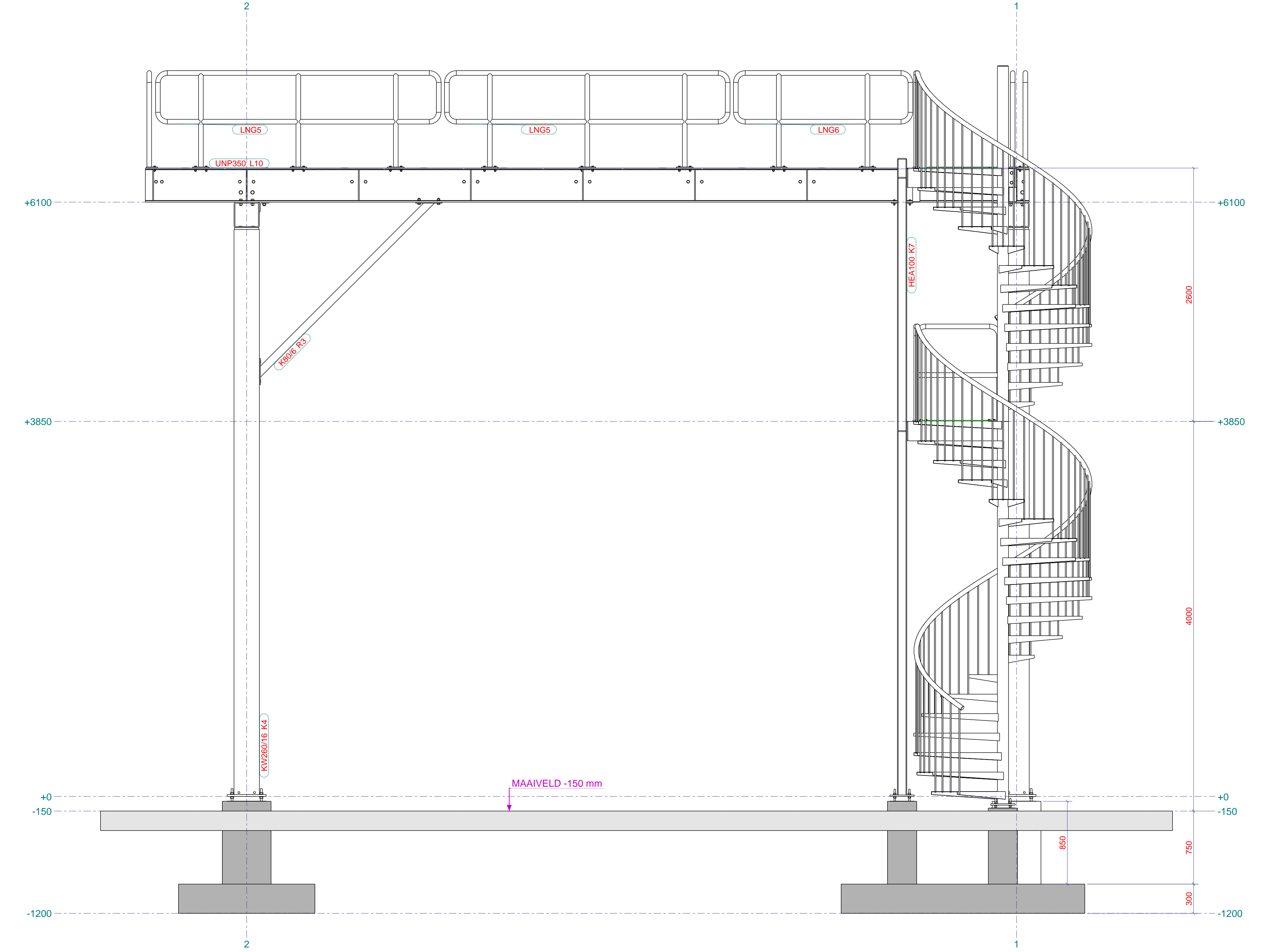
Achteraanzicht 1:25
