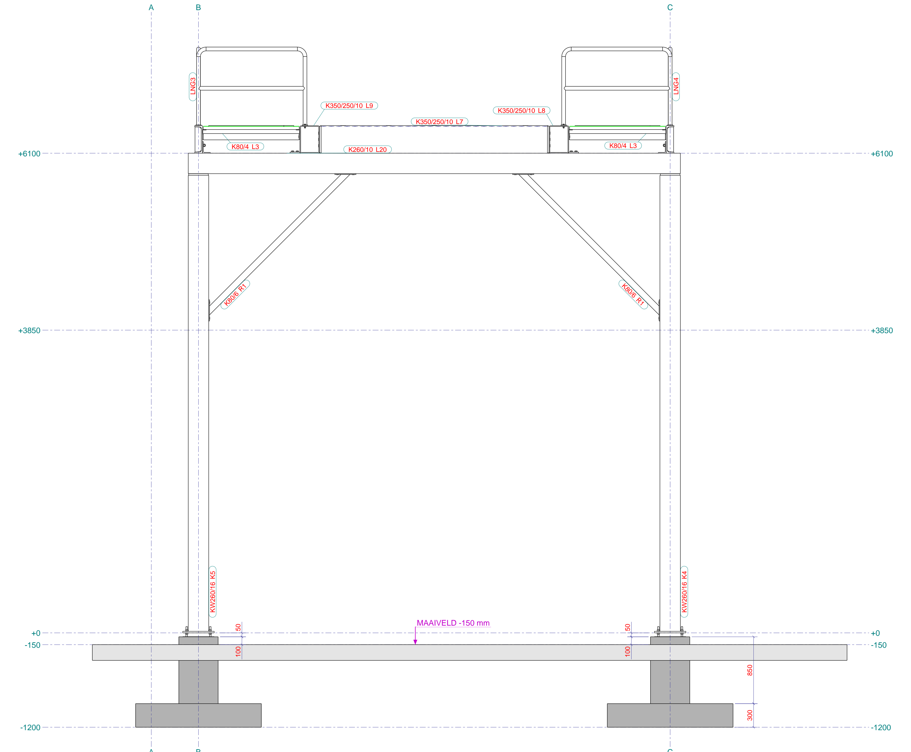
Rechter aanzicht 1:25
