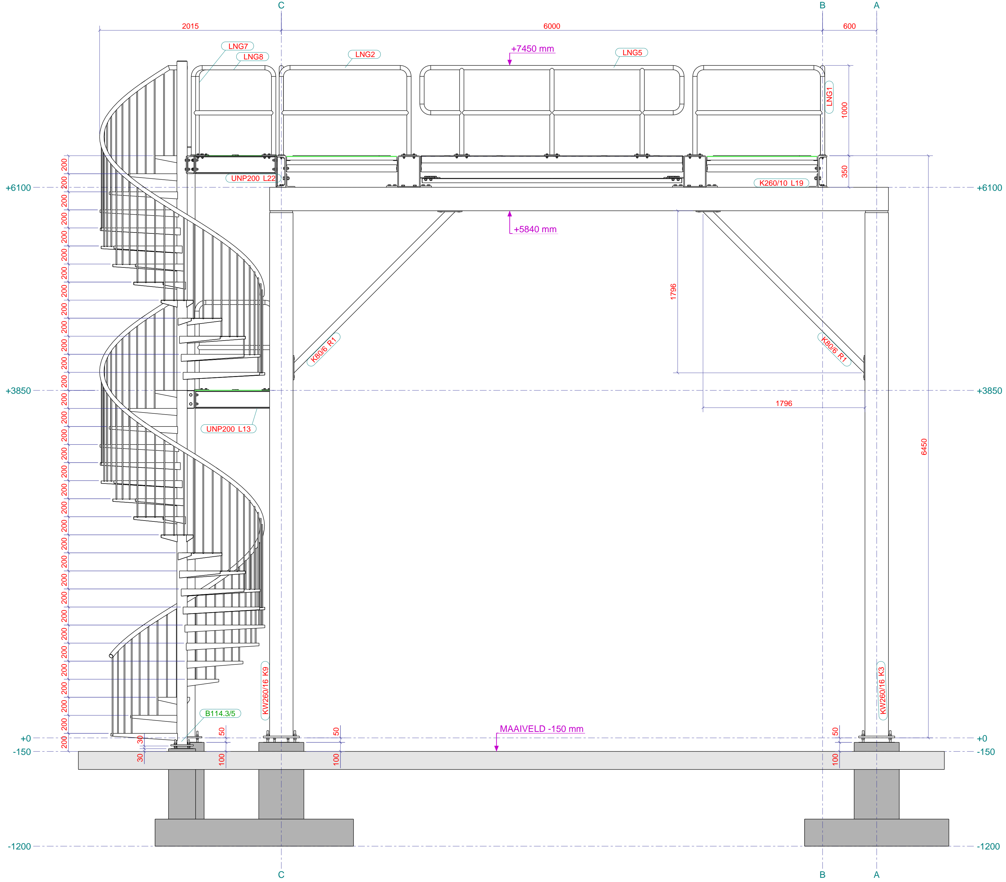
Linker aanzicht 1:25
