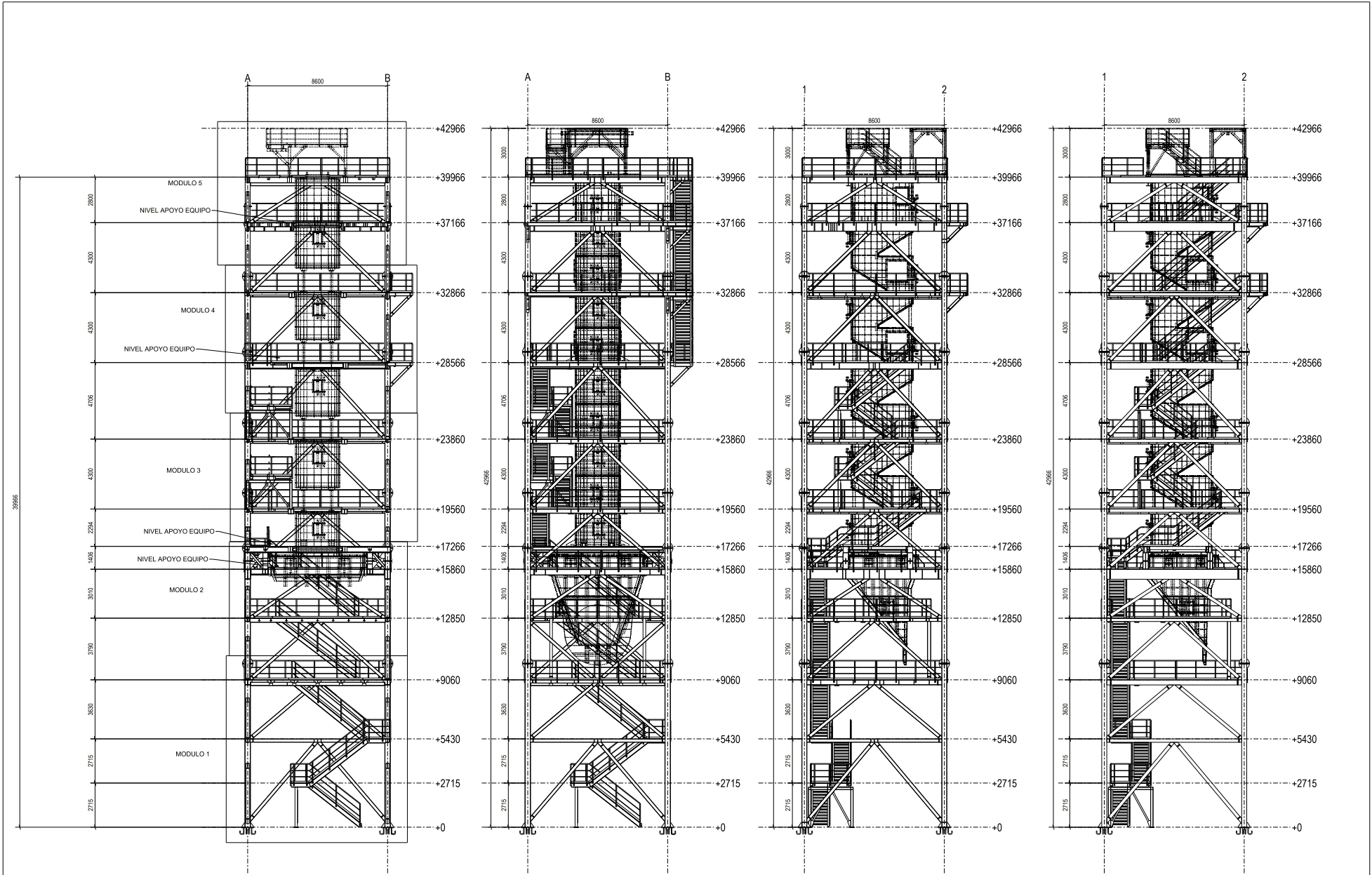
ALINEACION 1 E: 1:100
