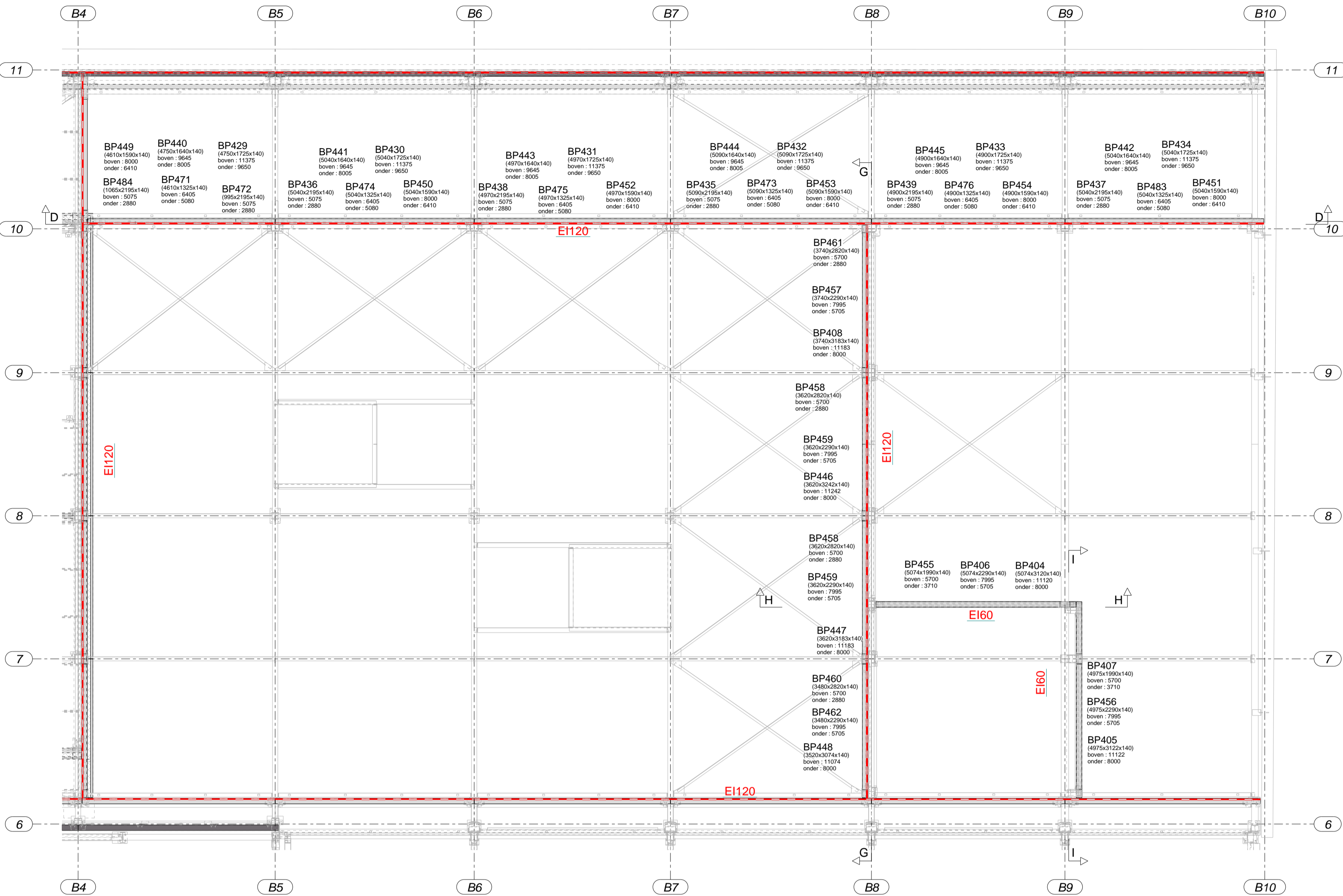
Bovenaanzicht +1 1:75
