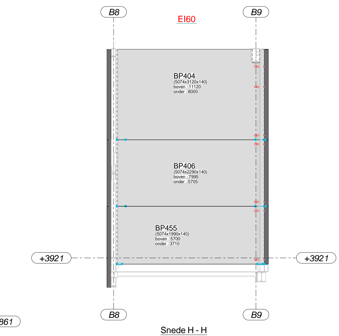
Sneded H - H 1:75
