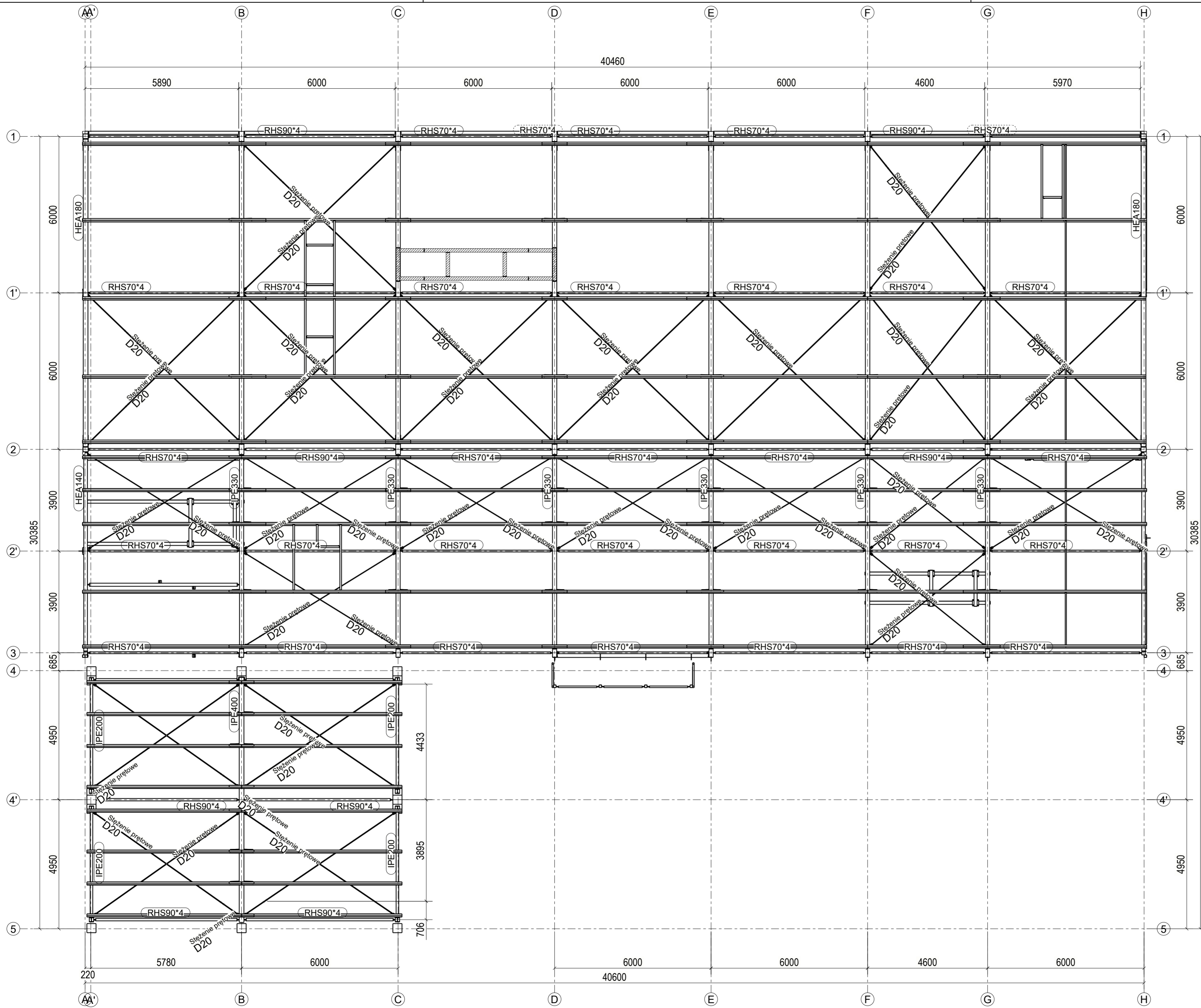
RZUT DACHU 1:100
