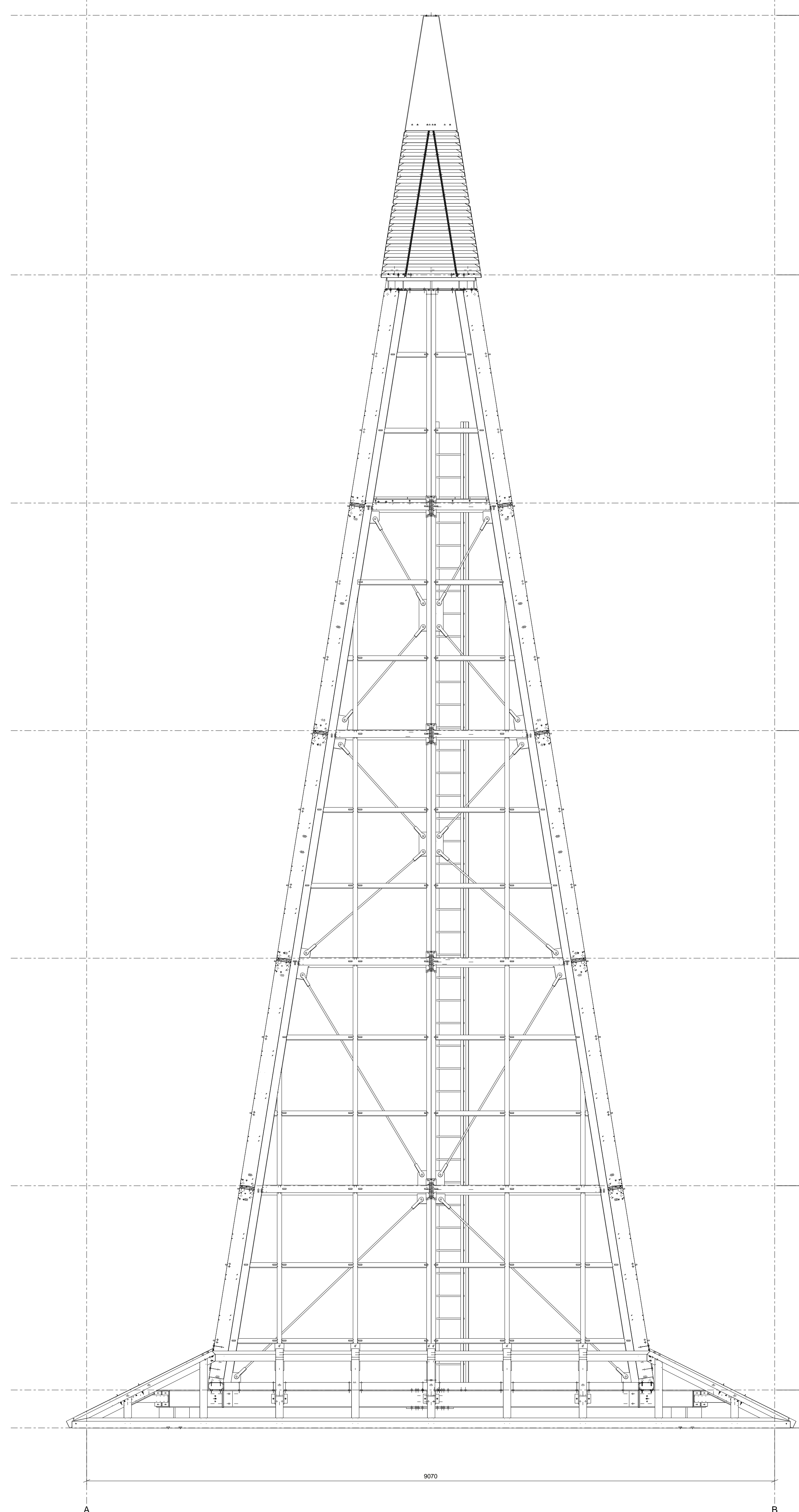
Aanzicht as 1 1:30
