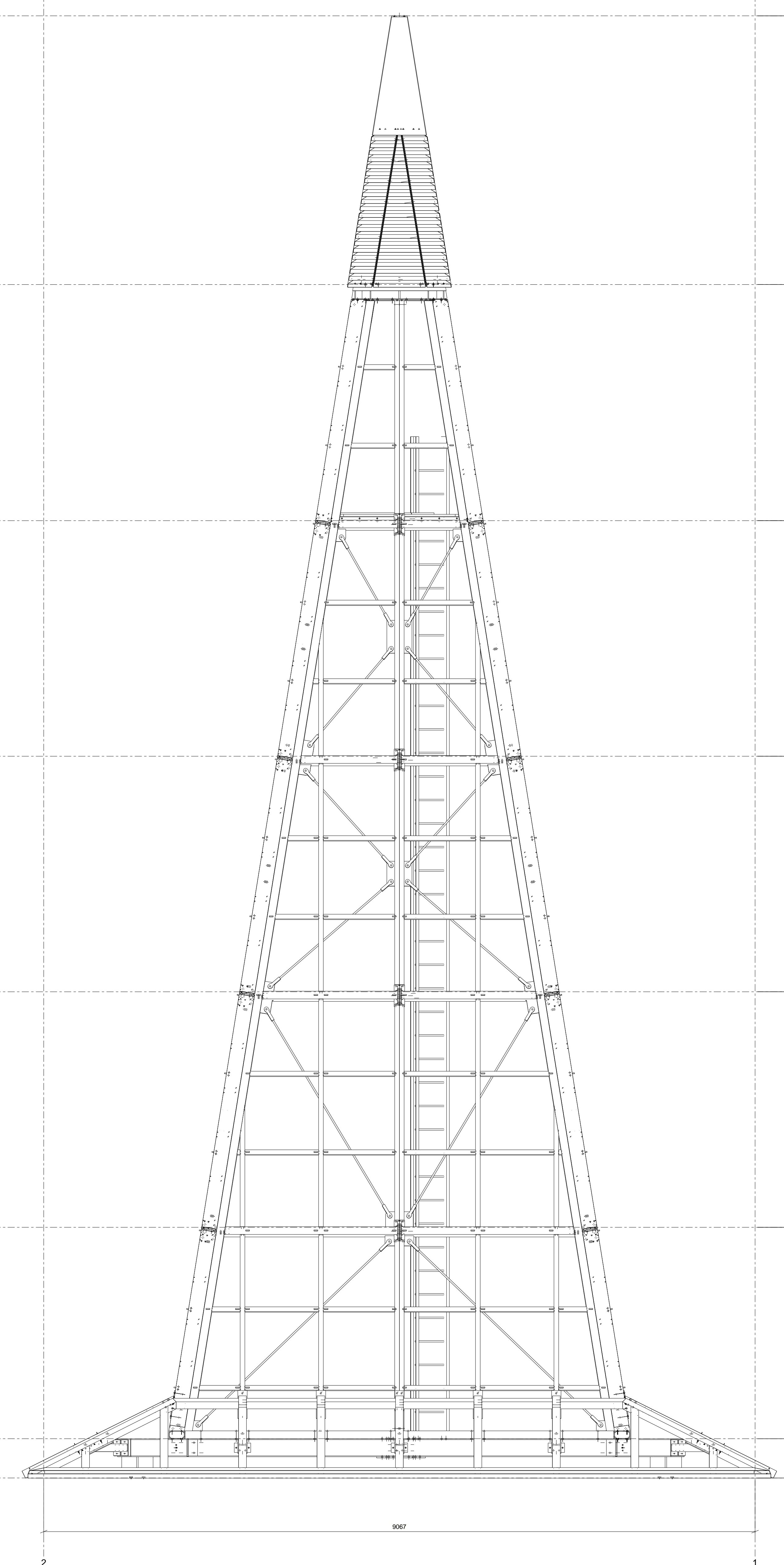
Aanzicht as A 1:30
